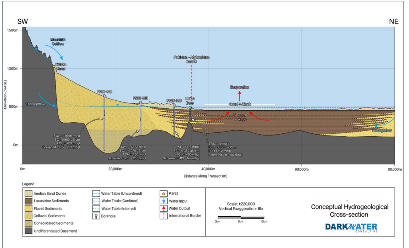
شکل 4 6: شمالی زمینی پانی کے حصے کے لیے اسکیمٹک تصوراتی ہائیڈرو جیولوجیکل کراس سیکشن صفحہ نمبر اکھاؤں پر ملاحظہ فرمائیں۔
