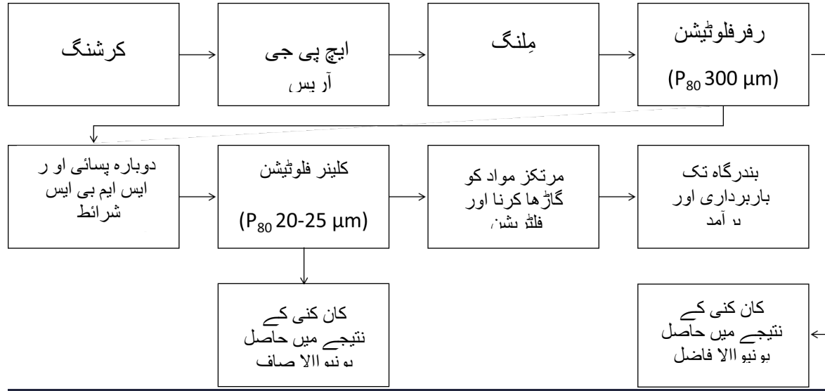
شکل 2-2 کچ دھات کی پراسسنگ کی فلو ڈائیگرام صفحہ نمبر تینیس پر ملاحظہ فرمائیں
