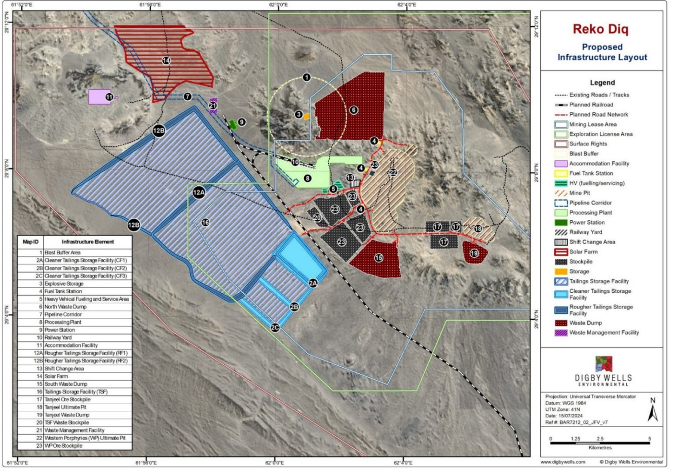
شکل 1-2 مجوزہ ریکوڈک مانن سائٹ کا خاکہ صفحہ نمبر بائیس پر ملاحظہ فرمائیں
