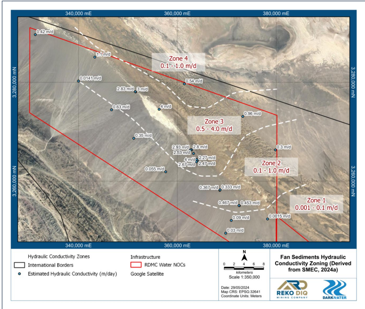
شکل 4-7: ہائیڈرولک کنڈکٹیویٹی زوننگ صفحہ نمبر ترین پر ملاحظہ فرمائیں 4.5.3.2.3 زیر زمین پانی کا معیار
