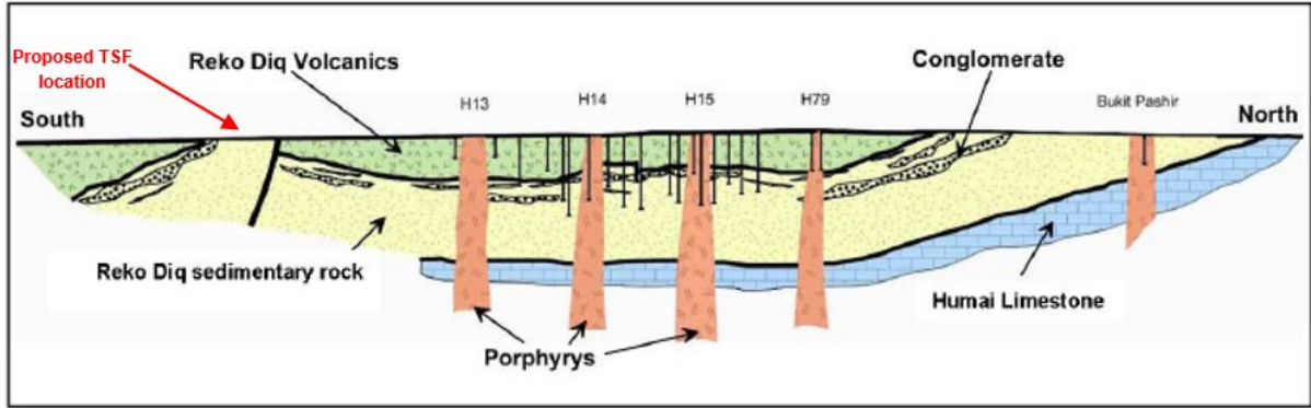
شکل 10 4: مغربی پورفیری کے ذریعے اسکیمیٹک جیولوجیکل کراس سیکشن صفحہ نمبر ستاون پر ملاحظہ
