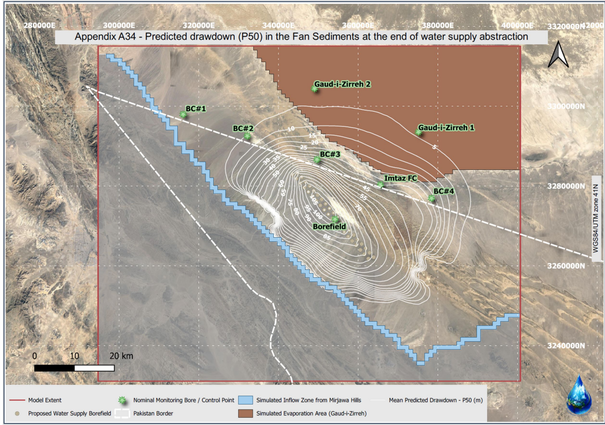
شکل 4 9: خلاصہ کے اختتام پر شمالی زمینی نظام میں P50 ڈرا ڈاؤن کی پیش گوئی (ڈارک واٹر، b2024) صفحہ نمبر چھپن پر ملاحظہ فرمائیں
