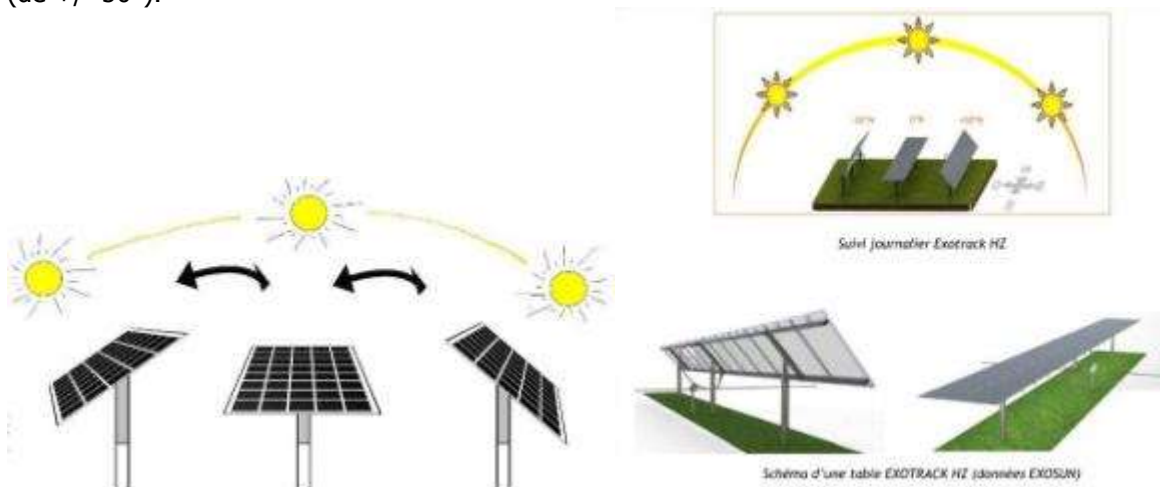
Figure 37 : Schéma de principe d'une installation photovoltaïque tracker un axe (source : EXOSUN)
