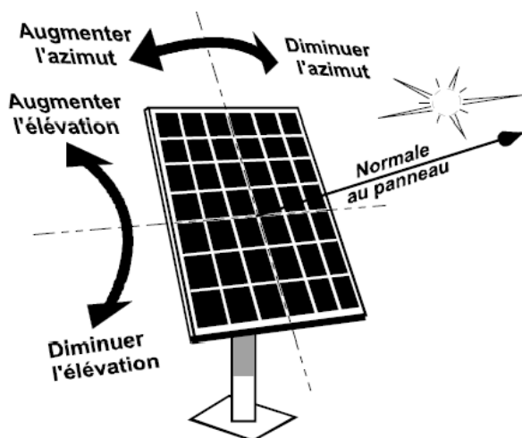
Figure 38 : Exemple de tracker 2 axes
