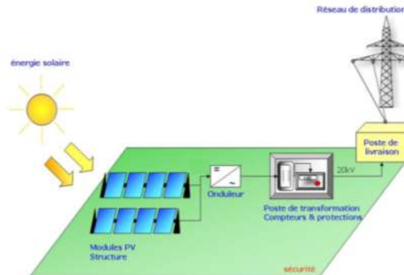
Figure 24 : Schéma de principe d'une installation photovoltaïque
