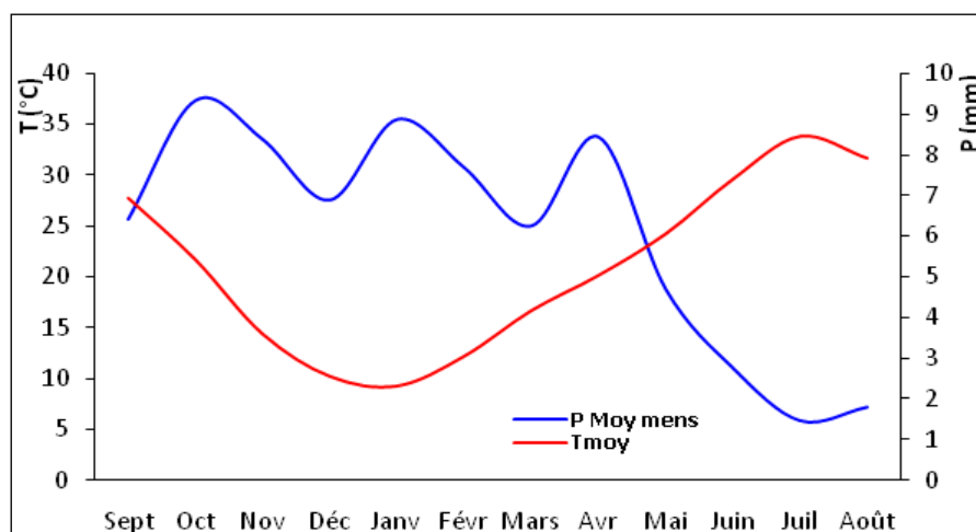
Figure 12 : Diagramme ombrothermique - Station : Radier Erfoud - Période : 1982-2009
