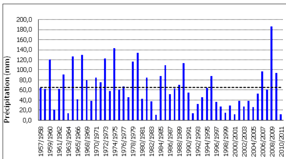
Figure 9 : Pluviométrie moyenne interannuelle - 1957/2011- Station Radier Erfoud
