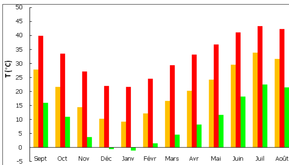
Figure 10 : Température moyenne mensuelle, minimale et maximale absolues (1982 - 2009) Station Radier Erfoud
