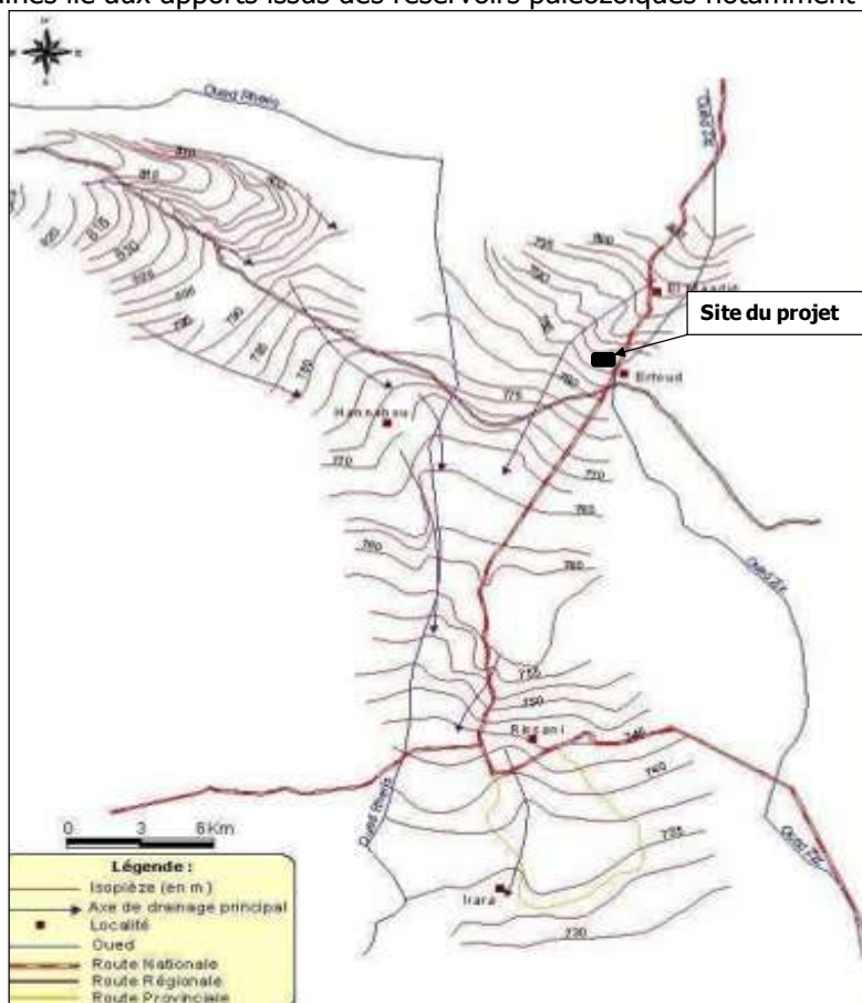
Figure 14 : piézométrie de la nappe de Tafilalt (Etude DRH GRZ/2006)
