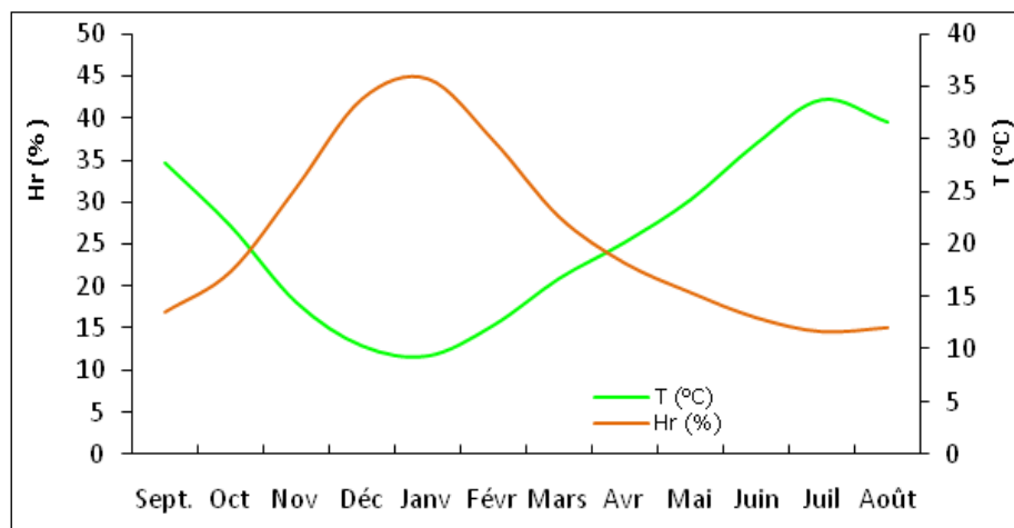
Figure 13 : Température moyenne interannuelle et hygrométrie de l'air Station Radier Erfoud - Période : 1996 – 2009
