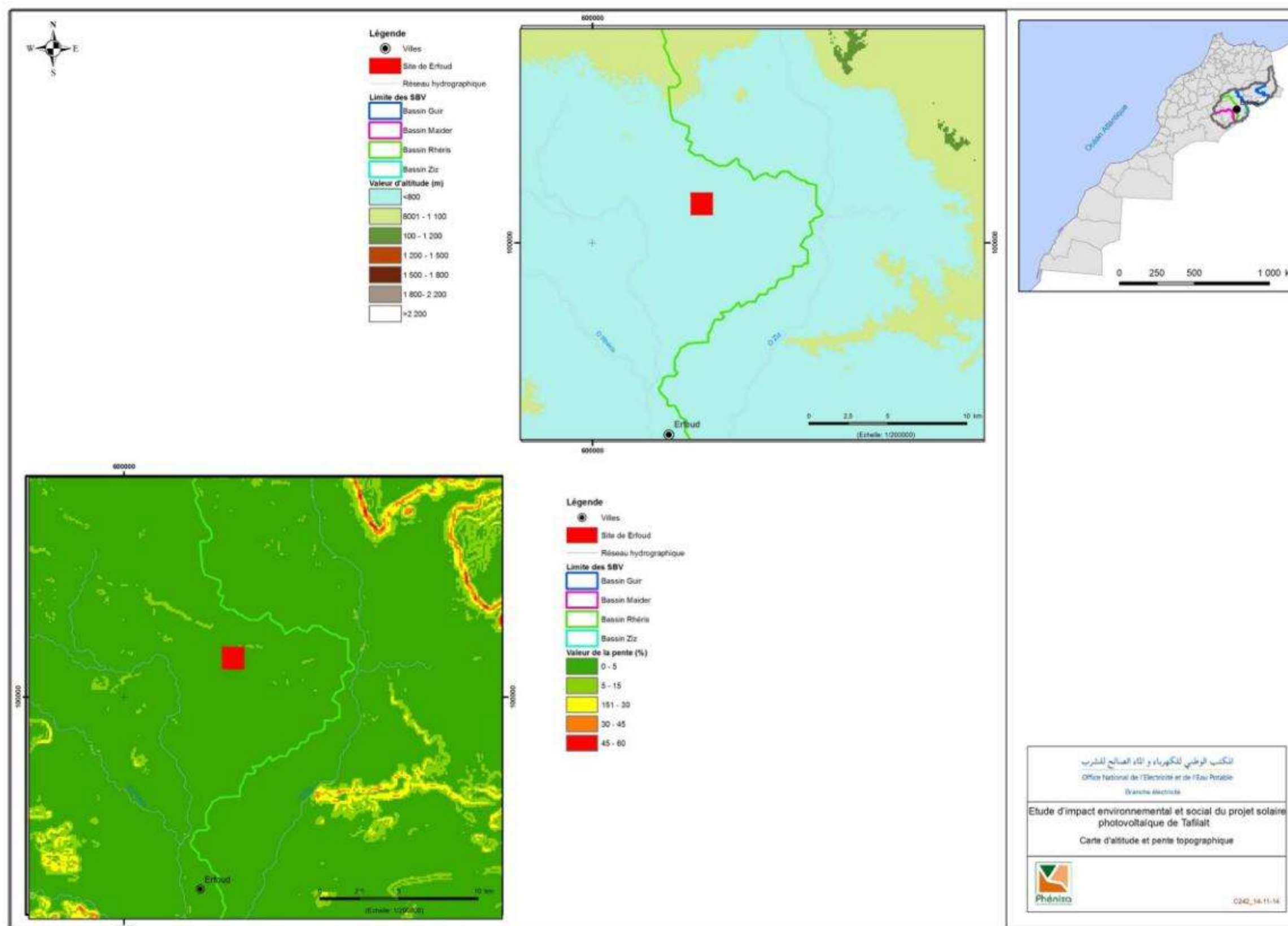
Figure 6 : Répartition spatiale de l'altitude et de la pente du site d'Erfoud
