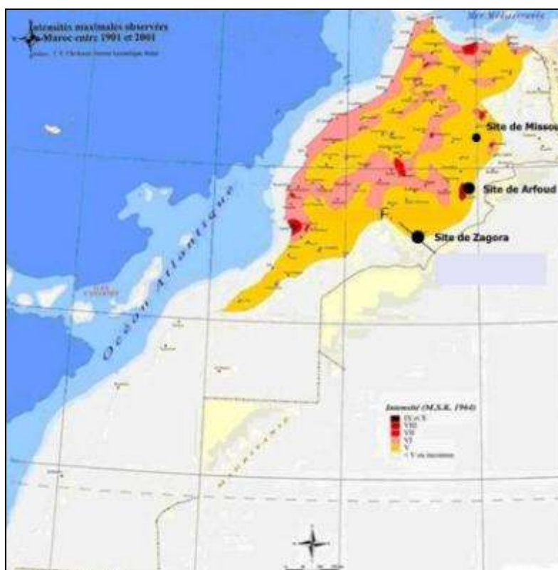
Figure 17 : Carte des intensités sismiques maximales ressenties : 1901-2001
