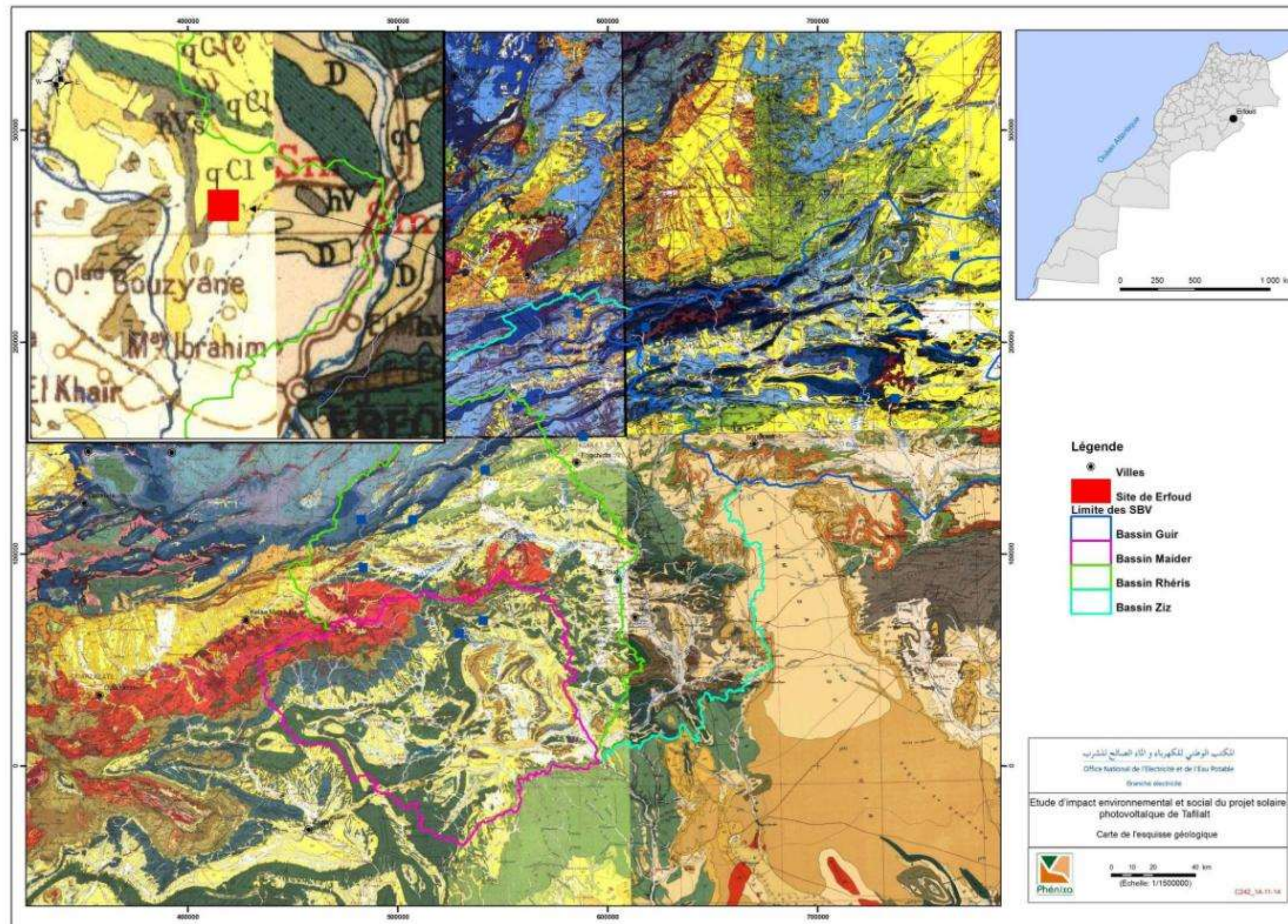
Figure 7 : Répartition spatiale des couches géologiques (Site d'Erfoud)
