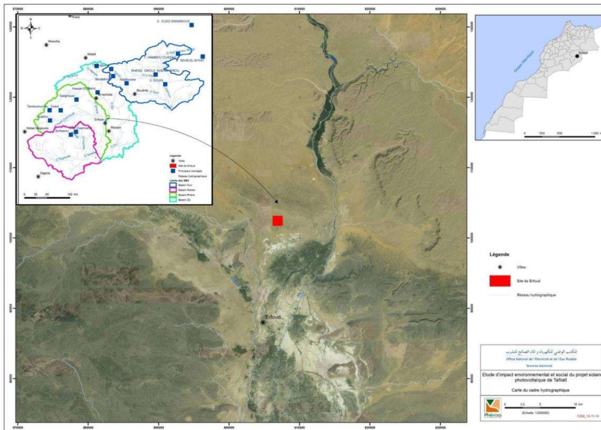
Figure 5 : Situation hydrographique du site d'Erfoud
