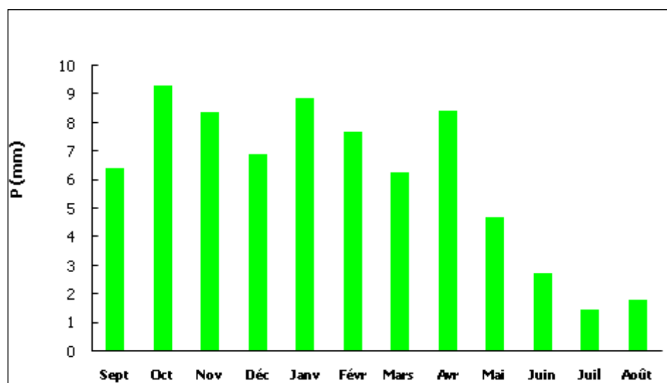
Figure 8 : Pluviométrie moyenne mensuelle - Période : 1957/2011
