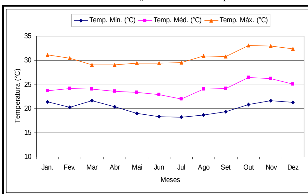
Gráfico 5.3 – Variação Anual da Temperatura
