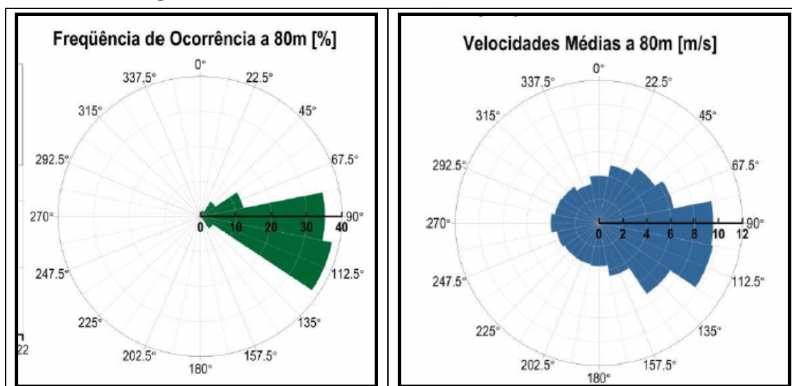
Figura 5.2 – Síntese das Medições de Ventos na Área
