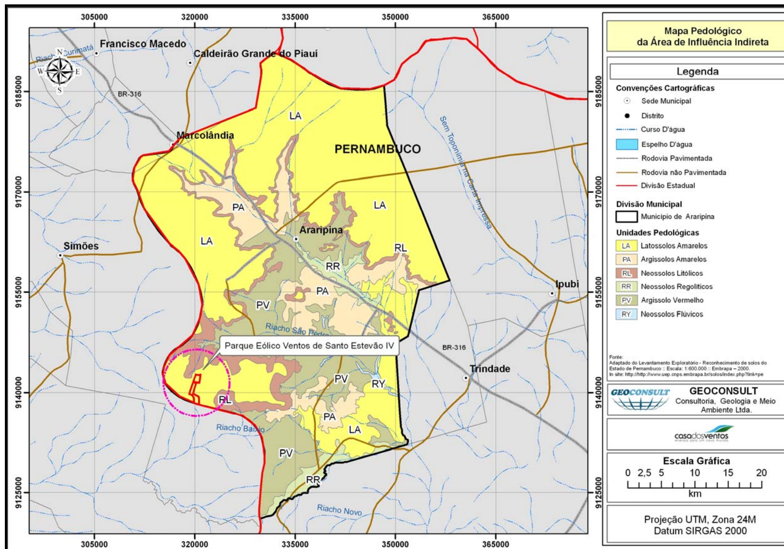
Figura 5.5 – Domínios Pedológicos do Município de Araripina
