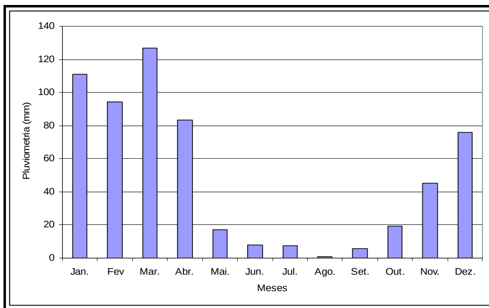
Gráfico 5.1 – Distribuição Pluviométrica ao Longo do Ano
