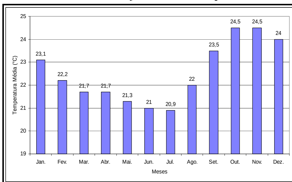
Gráfico 5.2 – Variação Mensal da Temperatura
