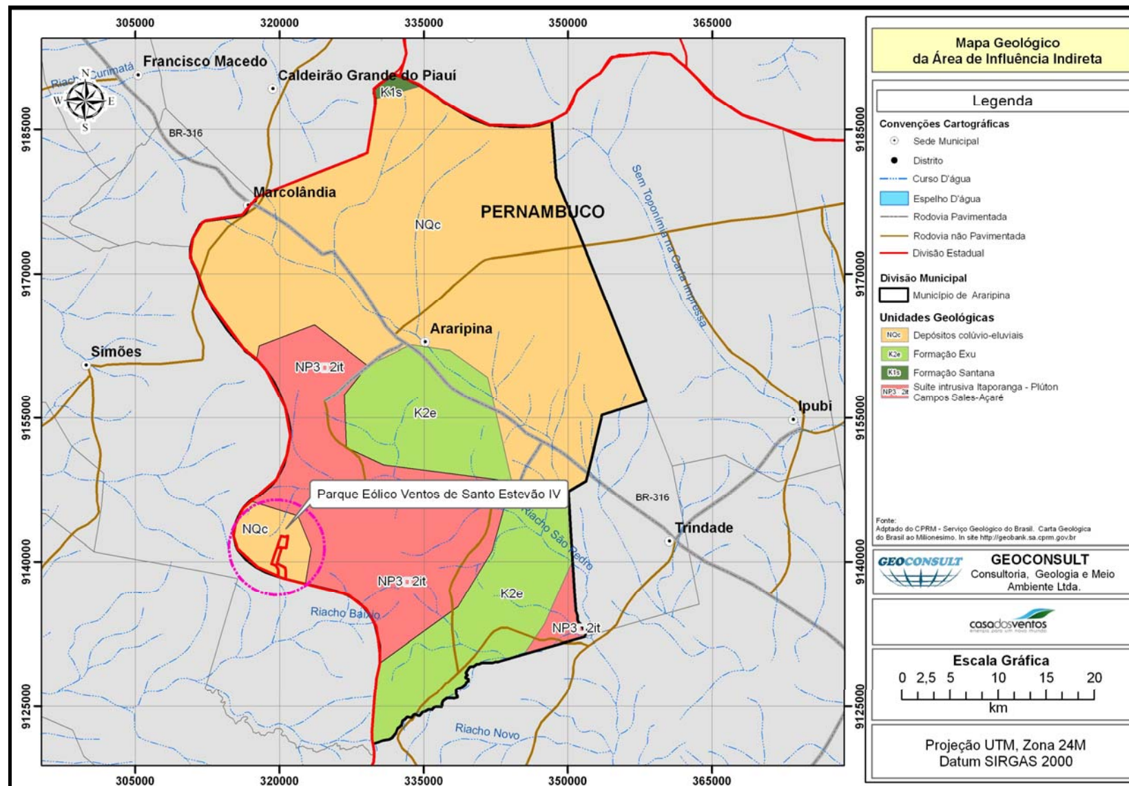
Figura 5.3 – Mapa Geológico da Área de Influência Indireta
