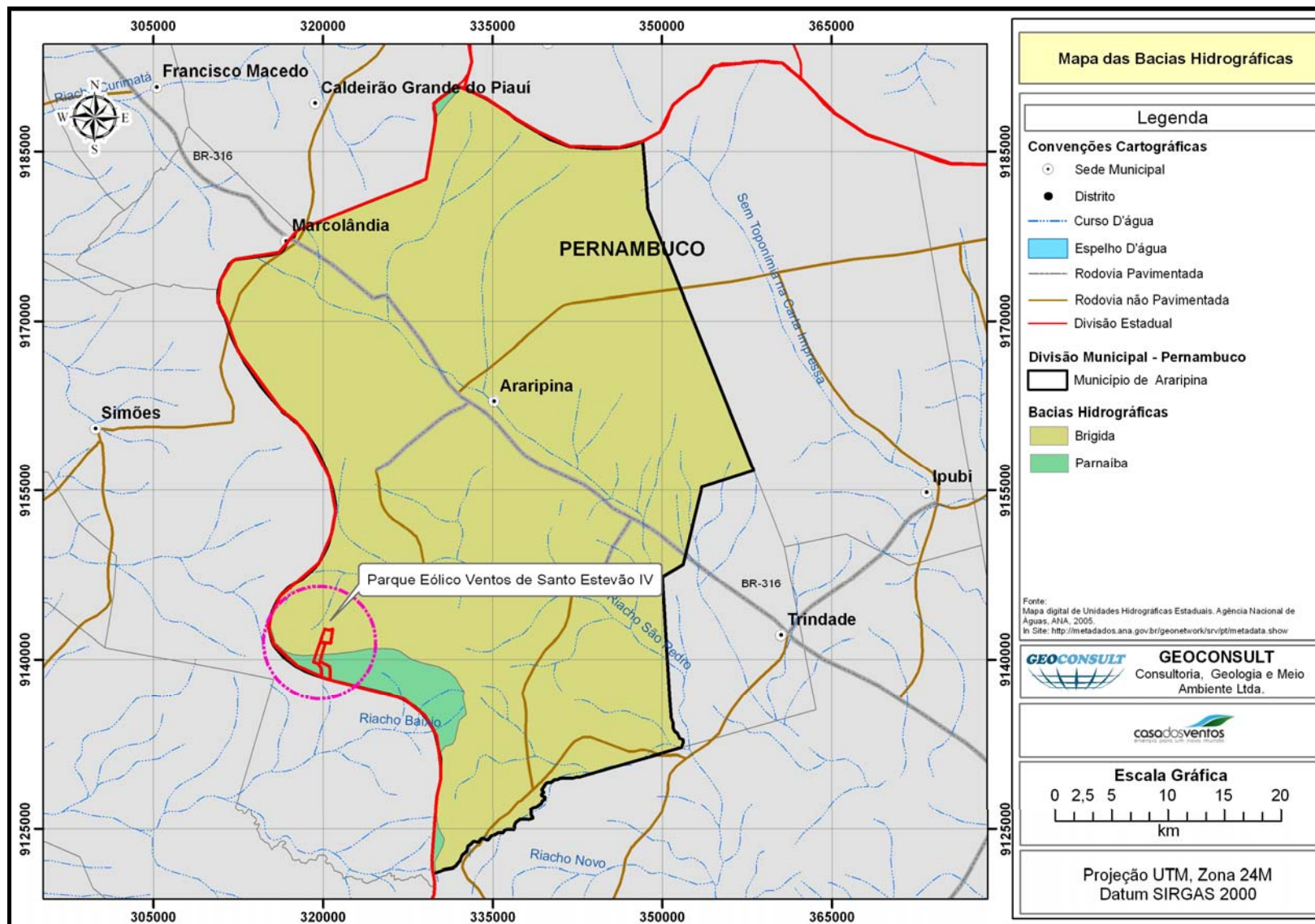
Figura 5.6 – Bacias Hidrográficas do Município de Araripina
