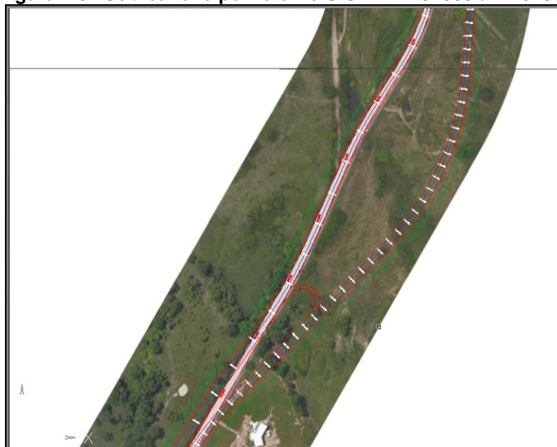
Figura 2-31 Sobreancho por retorno S-S. PR 125+800 al 126+500
