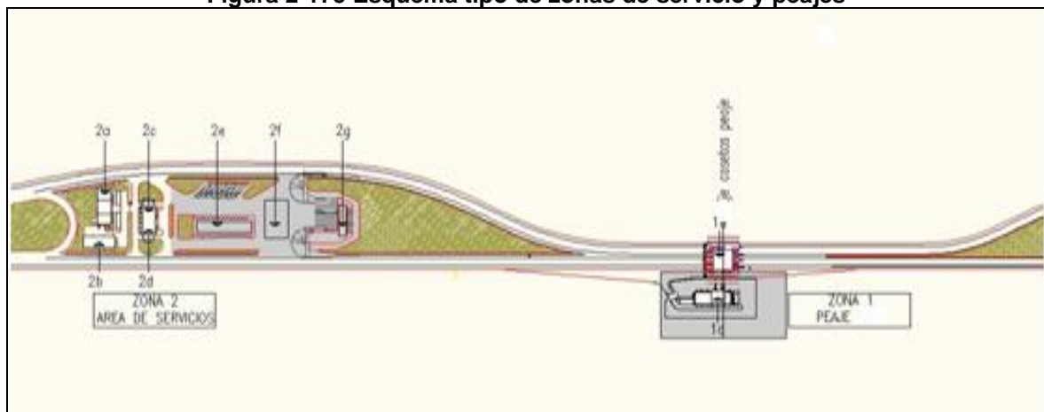
Figura 2-175 Esquema tipo de zonas de servicio y peajes
