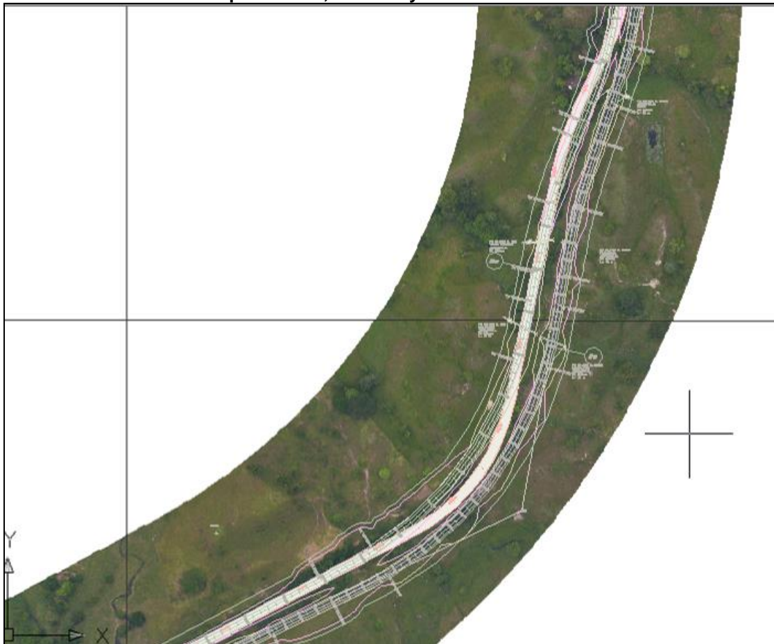
Figura 2-11 Sobrecancho por diseño geométrico PR 82+220 a PR 83+400, ancho máximo de separador 24,3 m Incluye realineamientos de la vía existente
