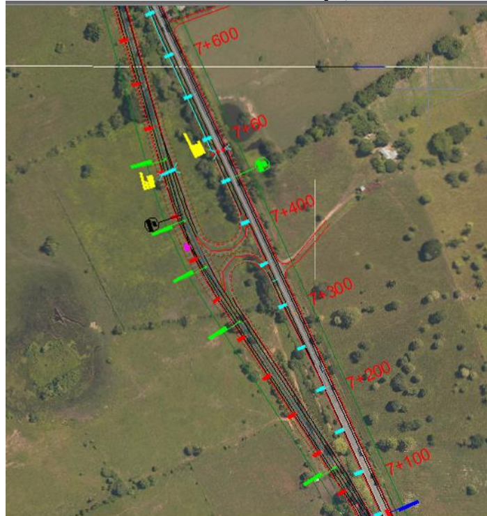
Figura 2-96 Retorno doble al sur de Pelaya, PR7+000 a PR7+850
