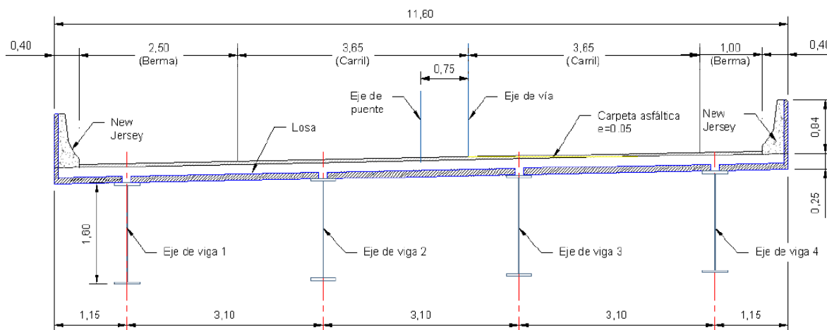
Sección transversal
