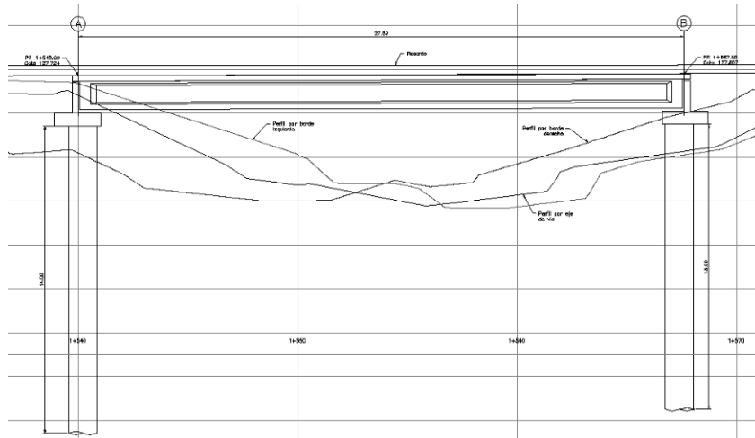
Perfil
