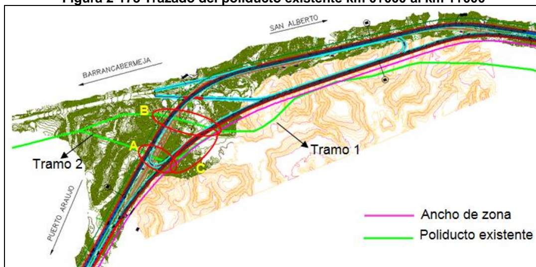
Figura 2-173 Trazado del poliducto existente km 0+000 al km 1+000
