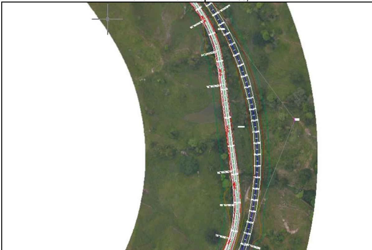
Figura 2-15 Sobrancho por diseño geométrico PR 89+870 al PR 90+310 Ancho máximo de separador 35,4
