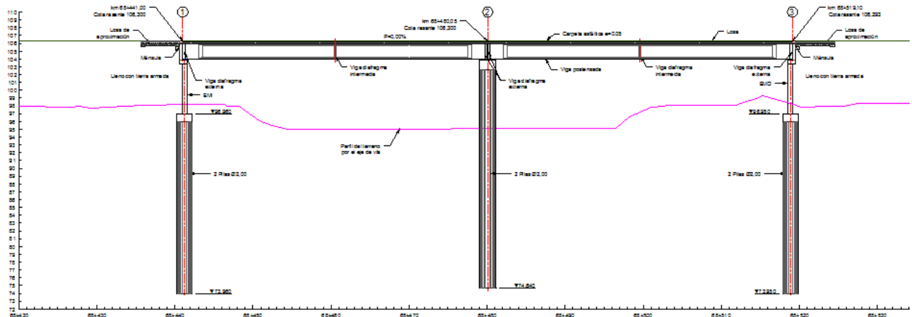
Perfil
