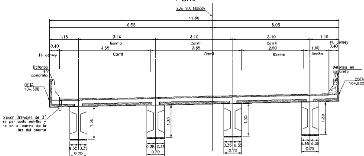
Sección Transversal
