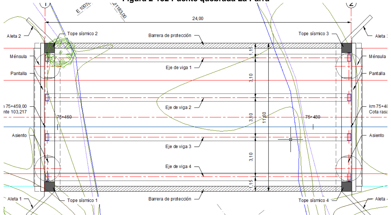
Planta
