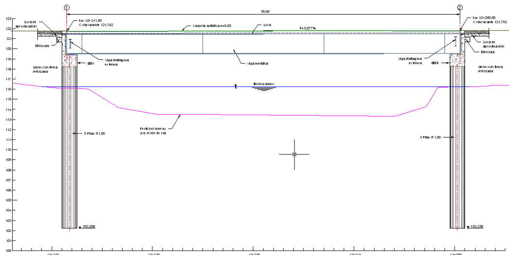
Perfil
