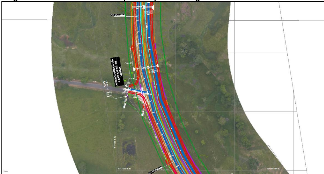
Figura 2-76 Sobrancho en el separador por diseño geométrico PR45+500 al PR45+750
