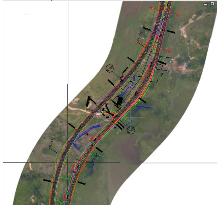
Figura 2-63 Sobreancho por retorno sencillo sur – sur PR 133+800 al PR134+860
