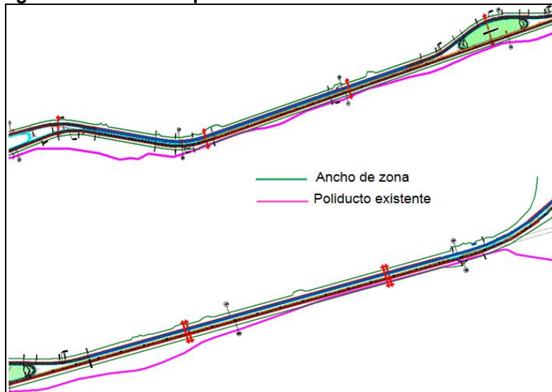
Figura 2-174 Trazado poliducto existente km 1+000 al km 6+000
