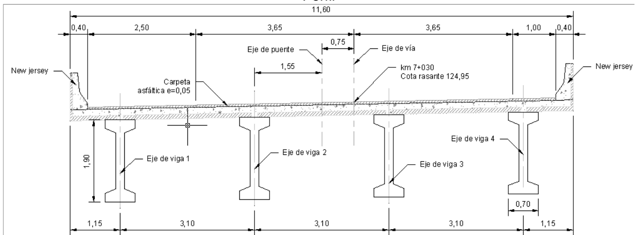
Sección Transversal
