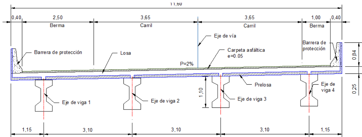
Sección transversal
