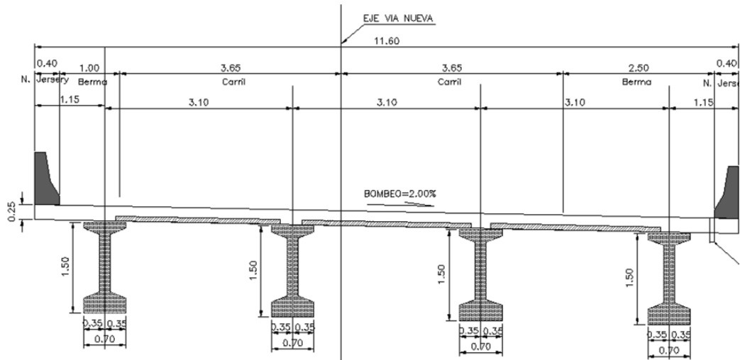
Sección Transversal
