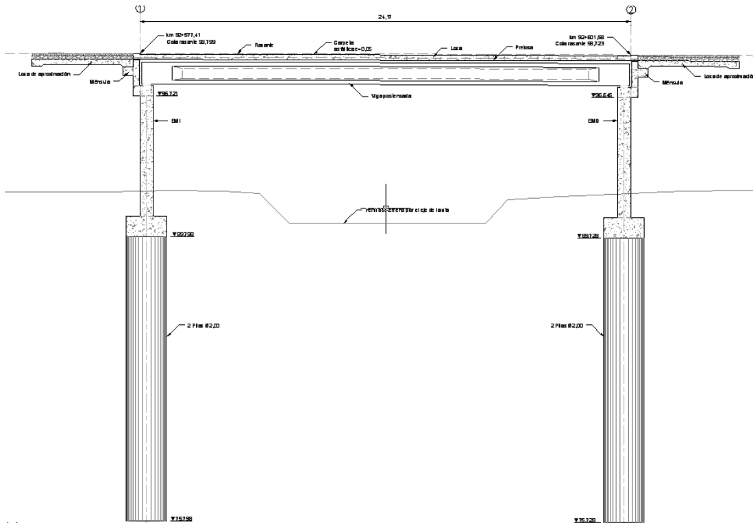
Perfil
