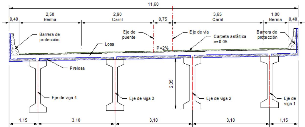
Sección transversal
