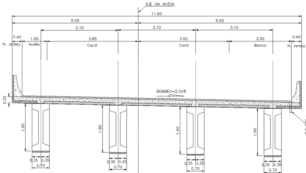
Sección transversal
