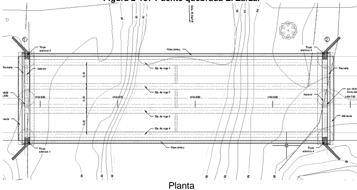
Figura 2-137 Puente quebrada El Zarzal
