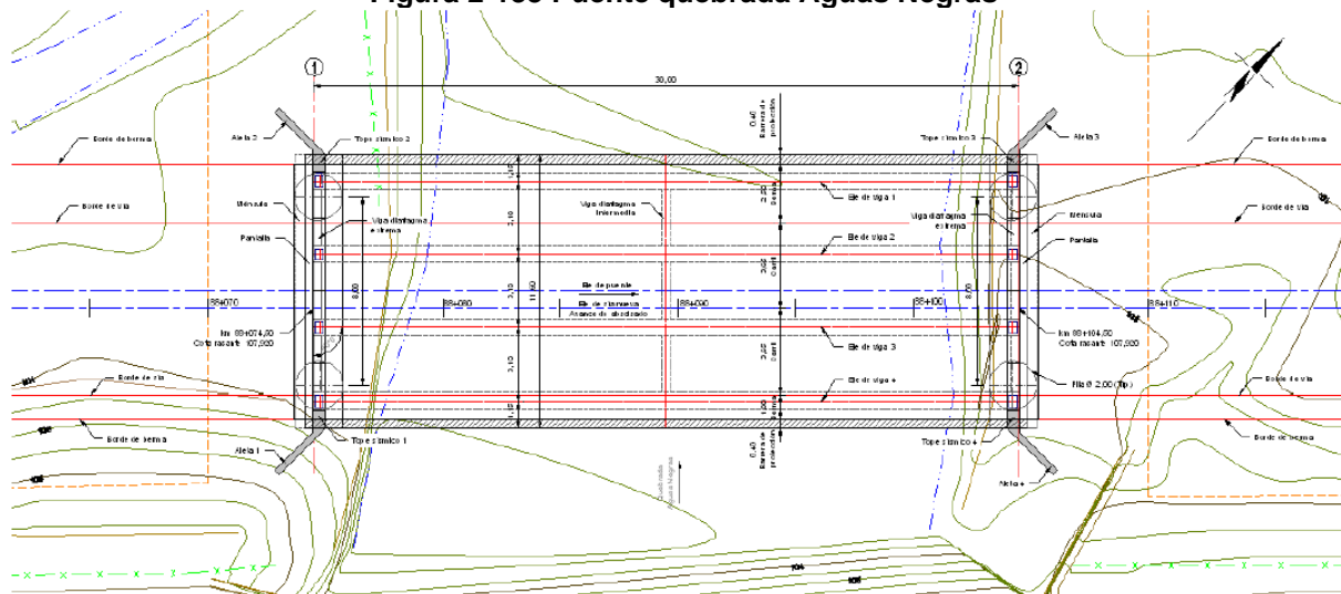
Planta
