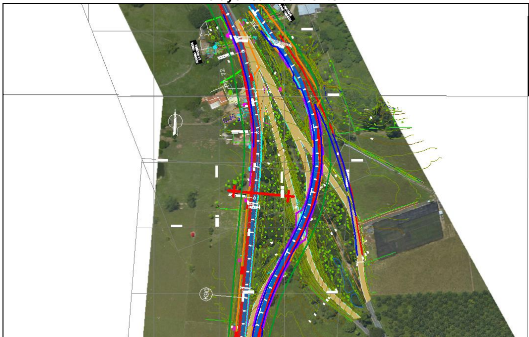
Figura 2-90 Intercambiador después de San Alberto PR 89+940 al PR90+600. Ancho aproximado 78,7. Incluye realineamiento
