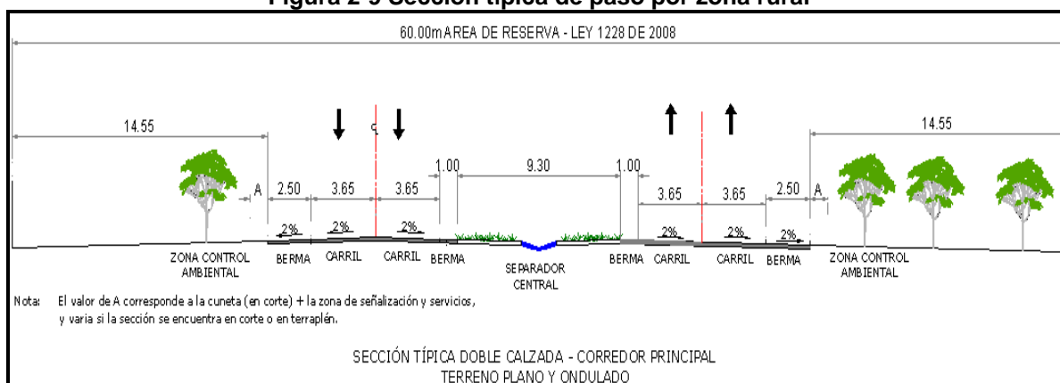
Figura 2-9 Sección típica de paso por zona rural
