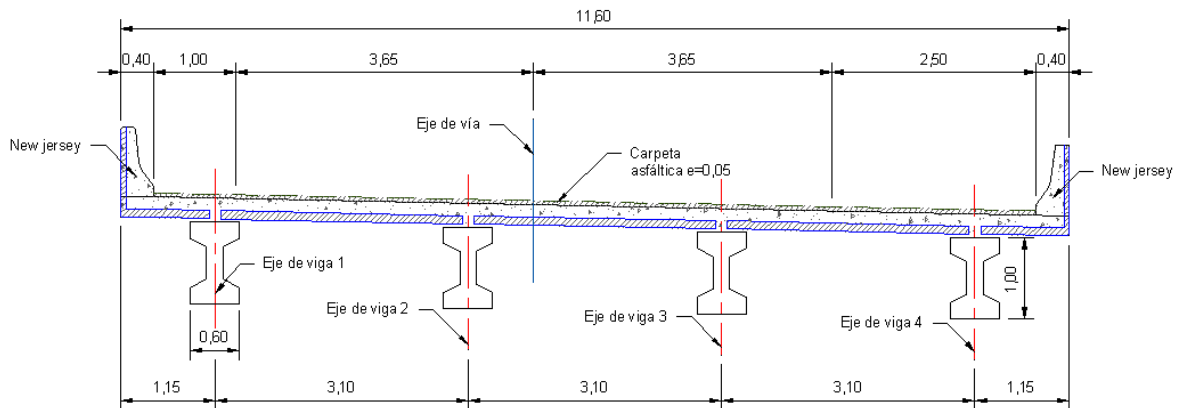
Sección Transversal
