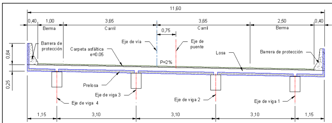
Sección Transversal
