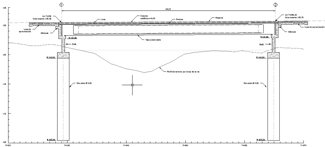
Perfil
