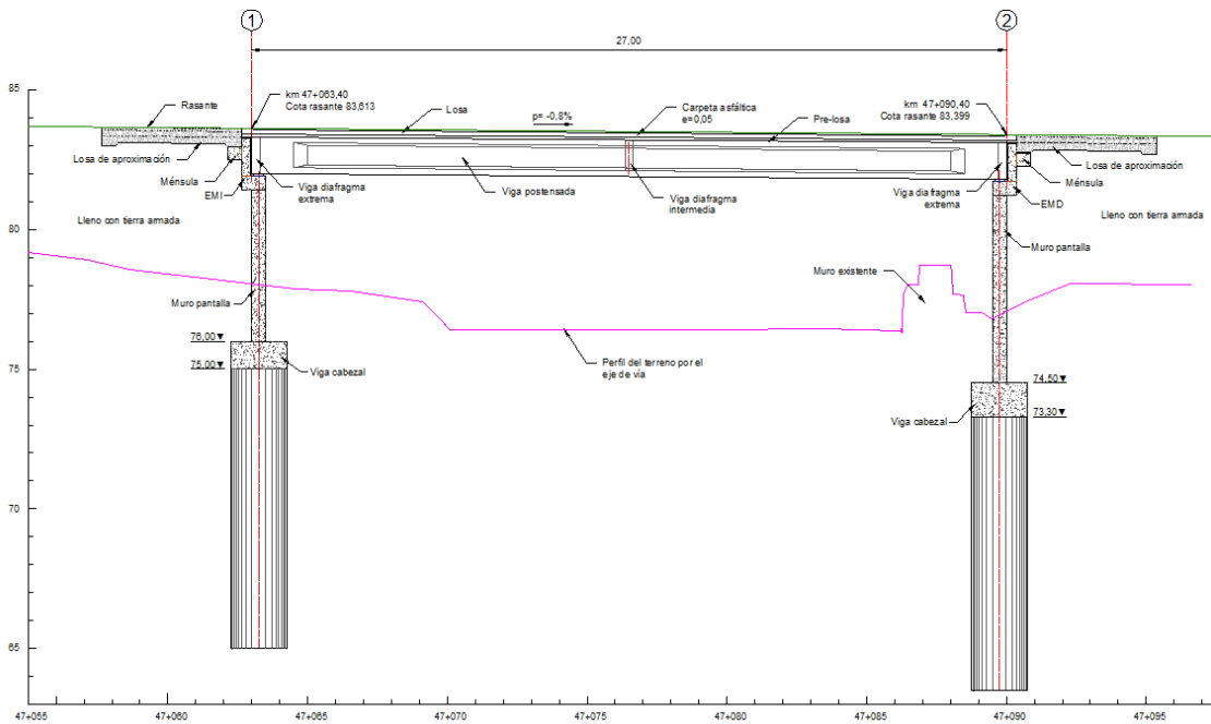
Perfil
