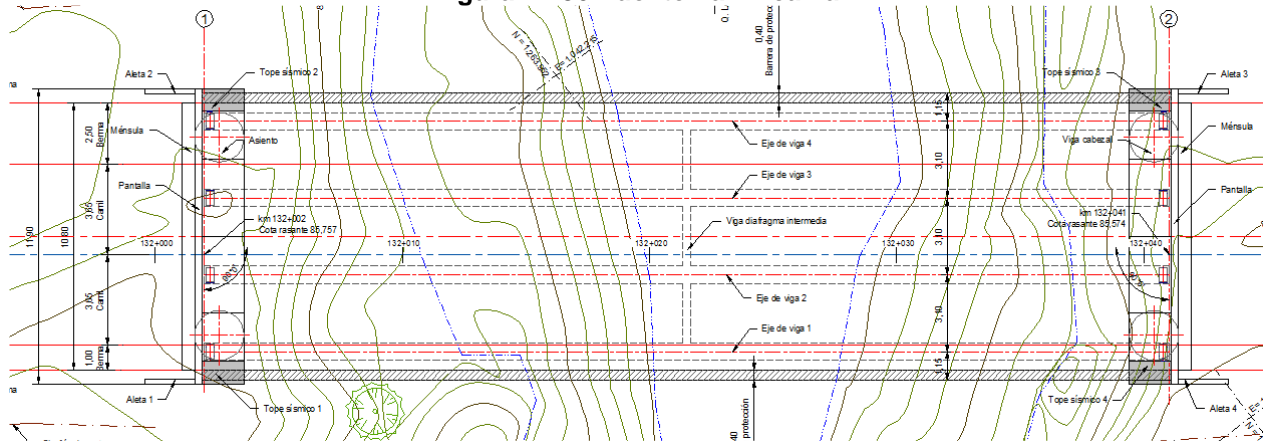
Planta
