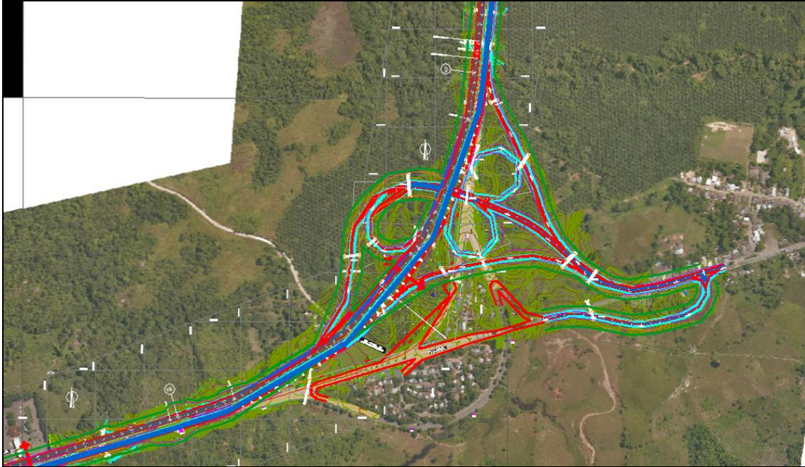
Figura 2-67 Intercambiador La Fortuna, incluye orejas para varios sentidos, interconectado este tramo con la vía a Bucaramanga. PR 6+060 al PR7+180
