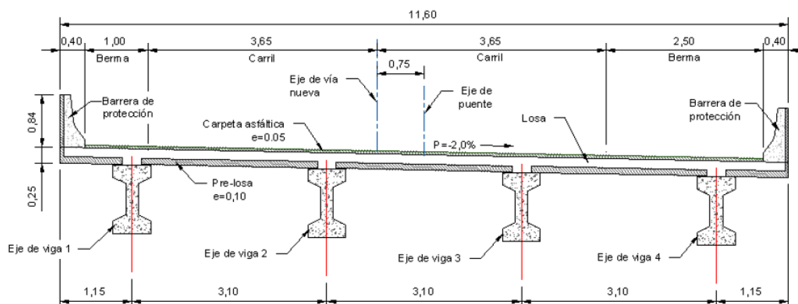
Sección Transversal
