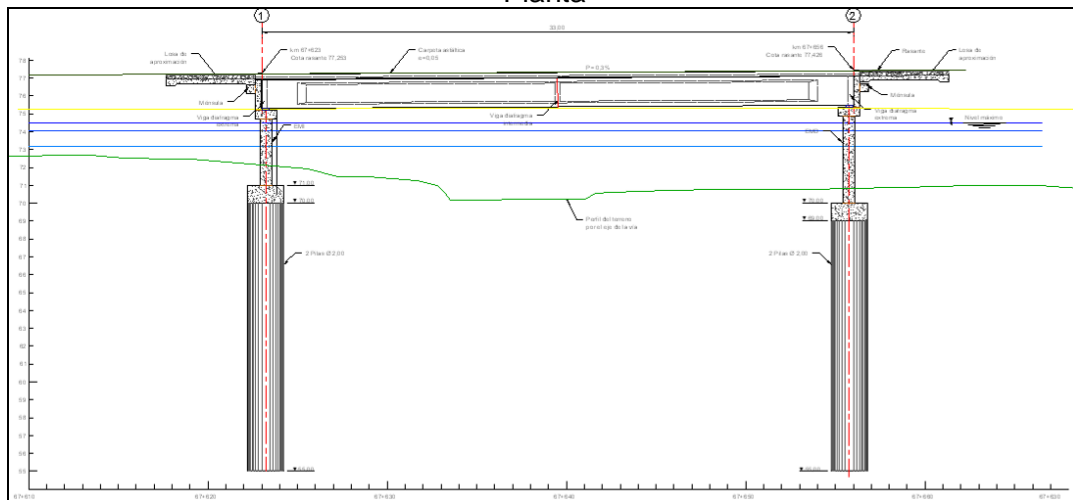
Perfil
