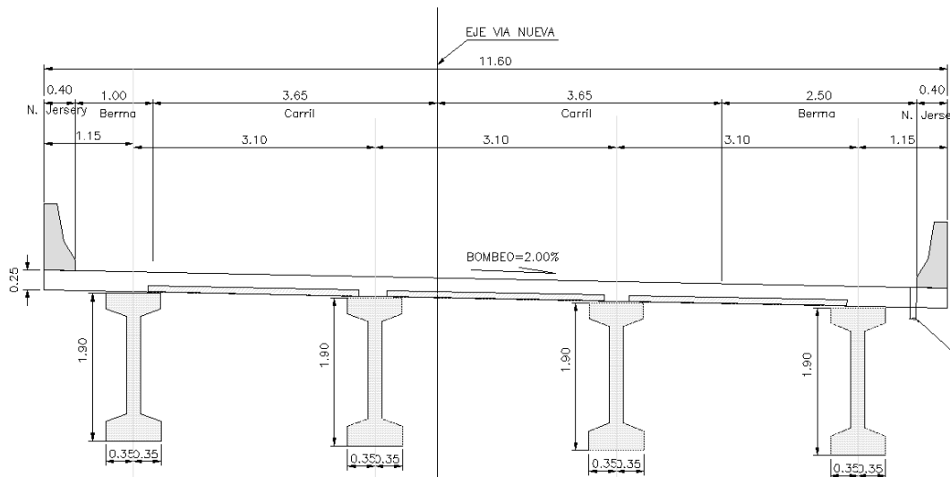
Sección Transversal
