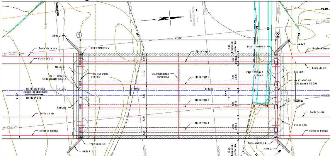
Planta
