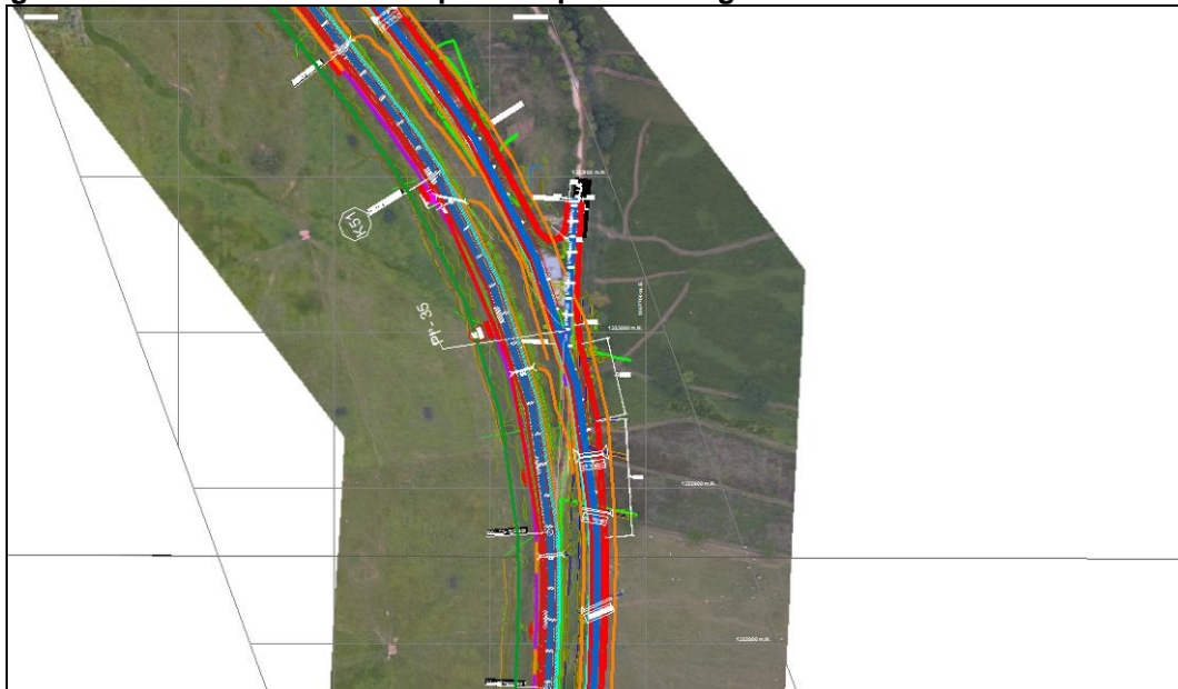
Figura 2-80 Sobreancho en el separador por diseño geométrico PR50+860 al PR51+110
