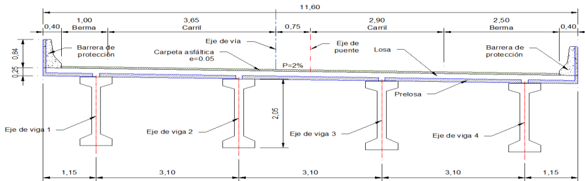
Sección transversal
