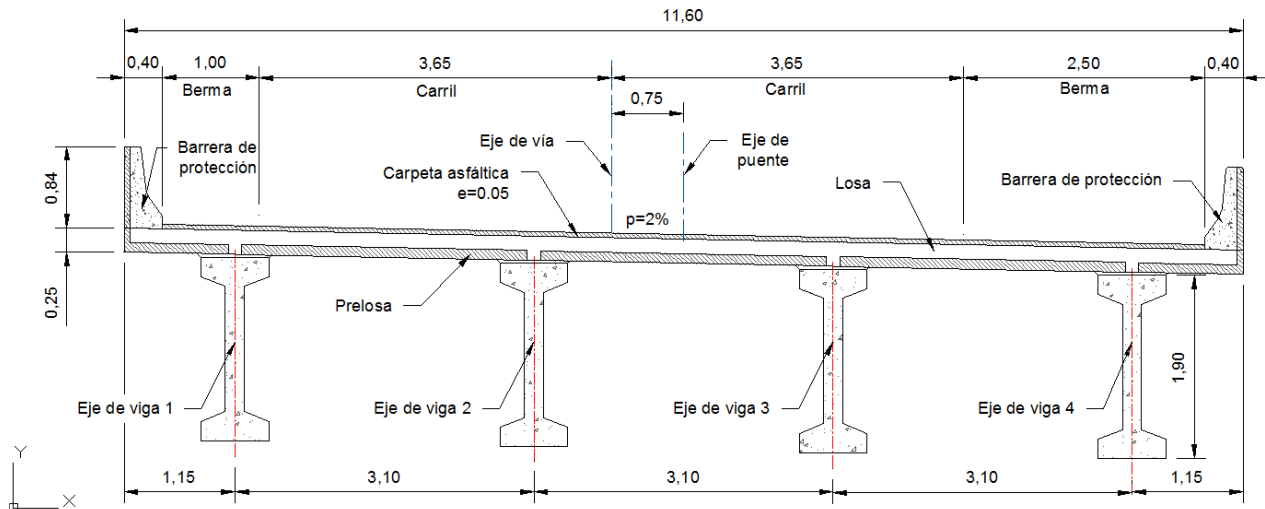
Sección transversal
