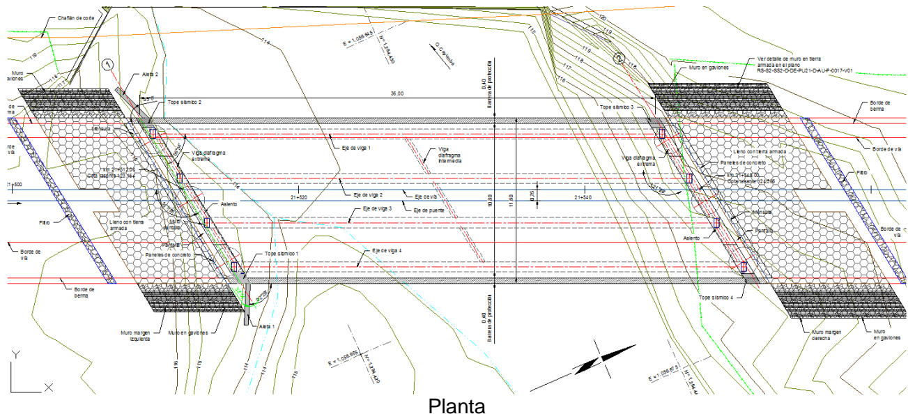
Figura 2-148 Puente 2 quebrada Cayumbita
