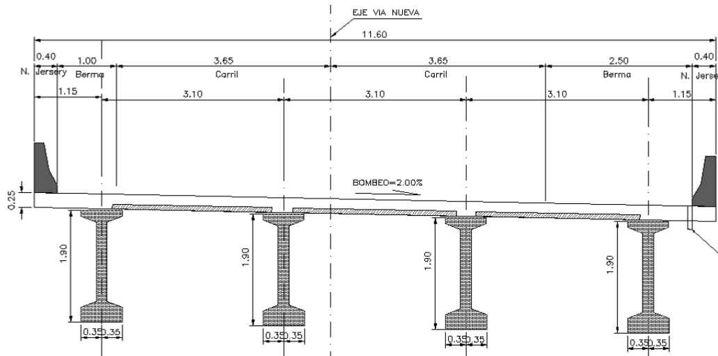
Sección Transversal
