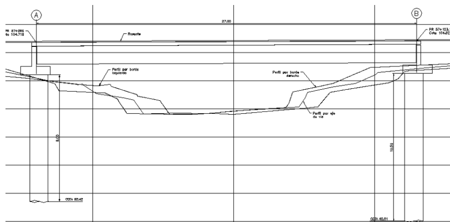
Perfil
