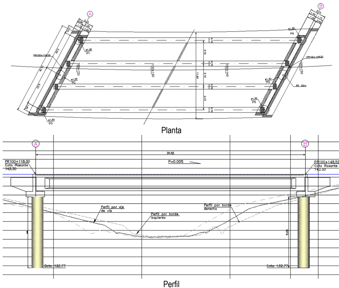
Figura 2-117 Puente Sacamujeres
