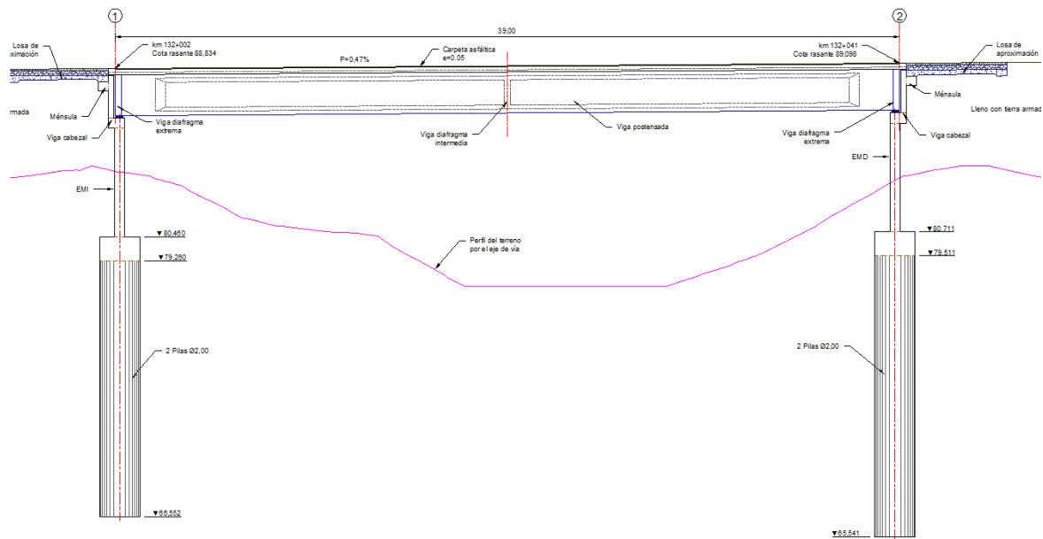
Perfil
