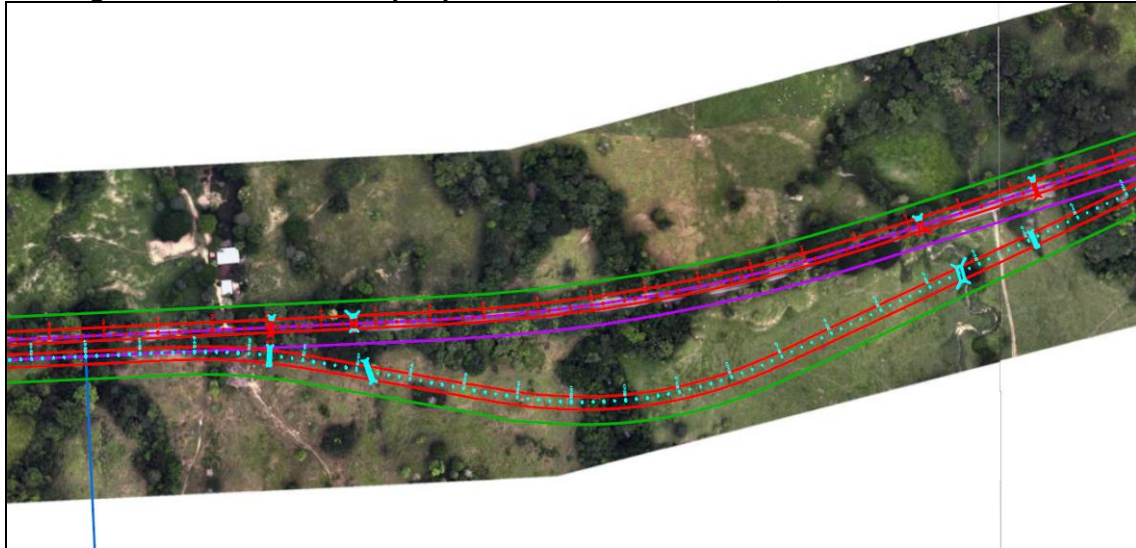
Figura 2-104 Sobreebanco por paso de la Quebrada Jairo, PR 46+300 a PR47+400
