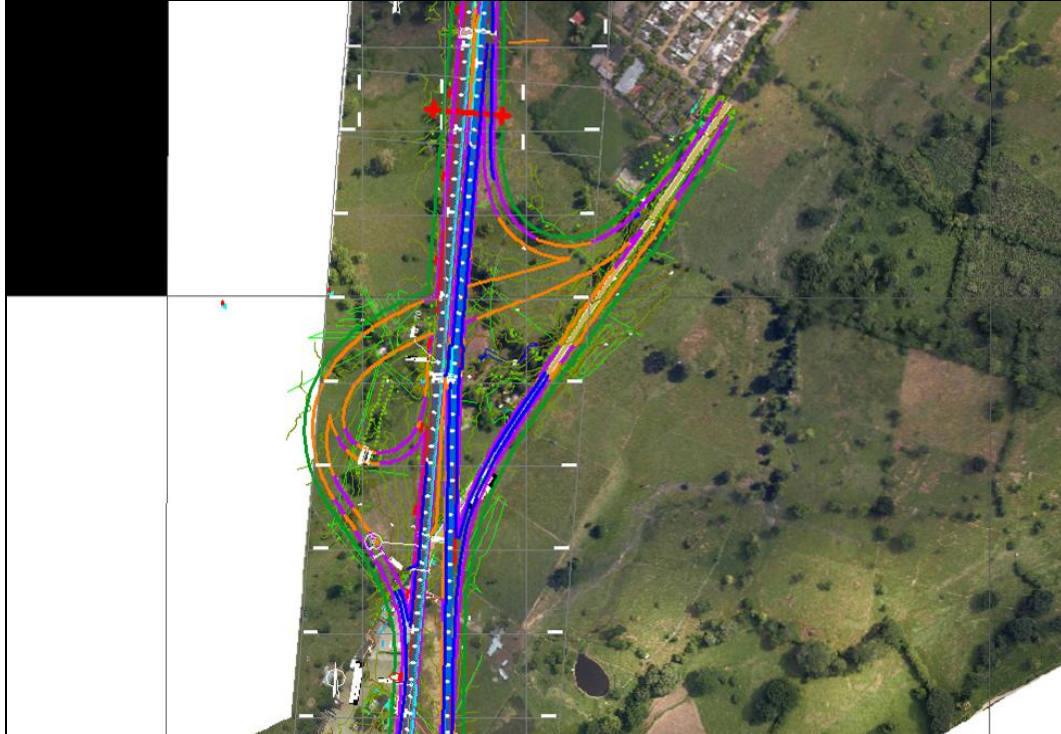
Figura 2-90 Intercambiador después de San Alberto PR 89+940 al PR90+600. Ancho aproximado 78,7. Incluye realineamiento
