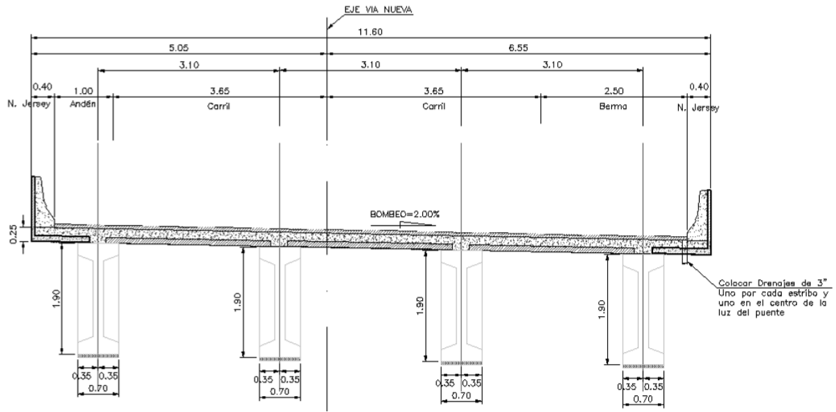
Sección transversal
