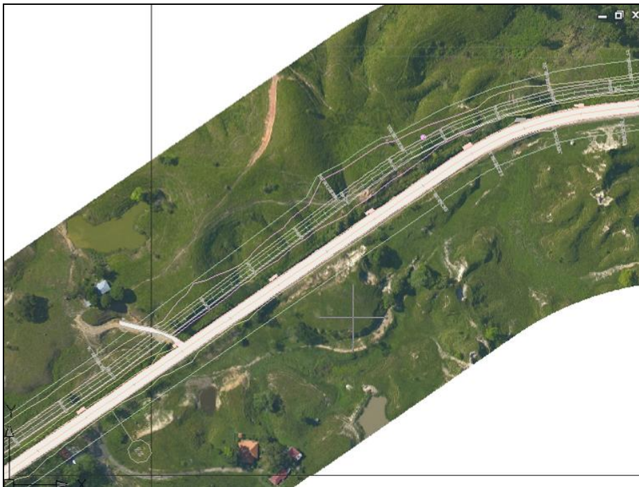
Figura 2-49 Sobreancho por diseño geométrico, PR58+050 al PR58+200, Ancho máximo del separador 19m
