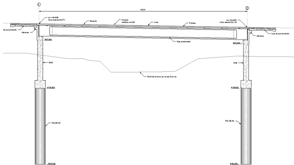
Perfil
