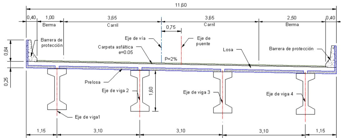
Sección Transversal
