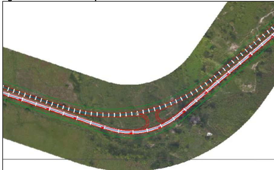
Figura 2-29 Sobreancho por retorno doble en PR 122+245 al PR 122+895,
