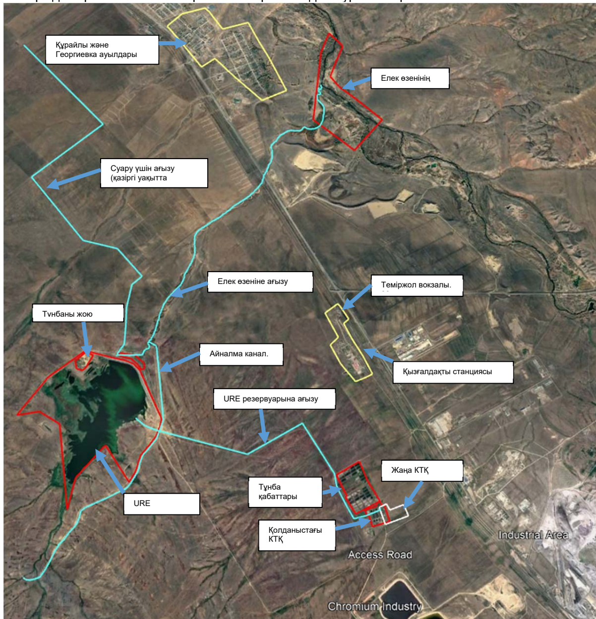
Сурет 2.2: ҚОӨСӘБ-ның ұсынылған КТҚ-ның зерттеу аймағы, негізінен қолданыстағы және жаңа КТҚ алаңдарынан, түнбаны тазарту алаңдарынан, КТҚ-дан URE резервуарынан, URE резервуарына және резервуардан Елек өзеніне, Елек өзеніне ағызуға арналған ашық арнадан тұрады. теңіз деңгейінен 500 м биіктікте және төгілу нүктесінен төмен-жобаға жақын орналасқан фермалар мен ауылдар (ең жақын ауылдар сары сызықтармен белгіленген). (Карта көзі: Google Earth)
