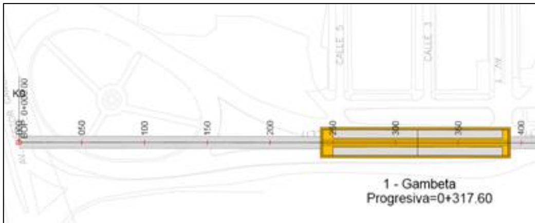
Figura 4-4 Espacio de aparcamiento de trenes después de estaciones terminales
