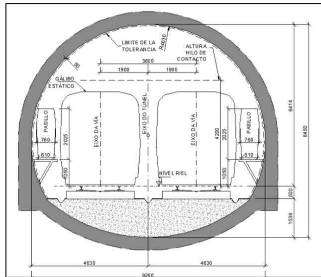
Figura 4-6. Sección en Caverna
