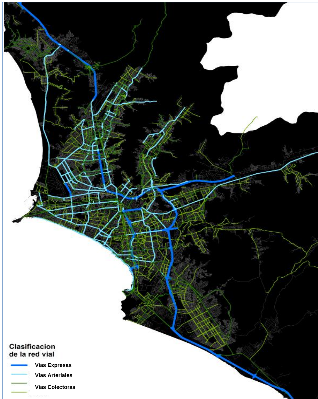
Figura 4-2 Clasificación de la red vial
