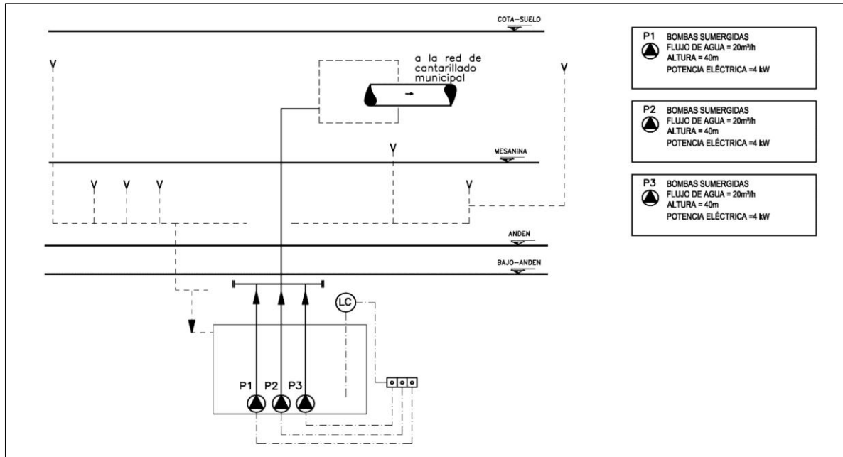
Figura 4-29 Sistema de Elevación de Aguas de Drenaje
