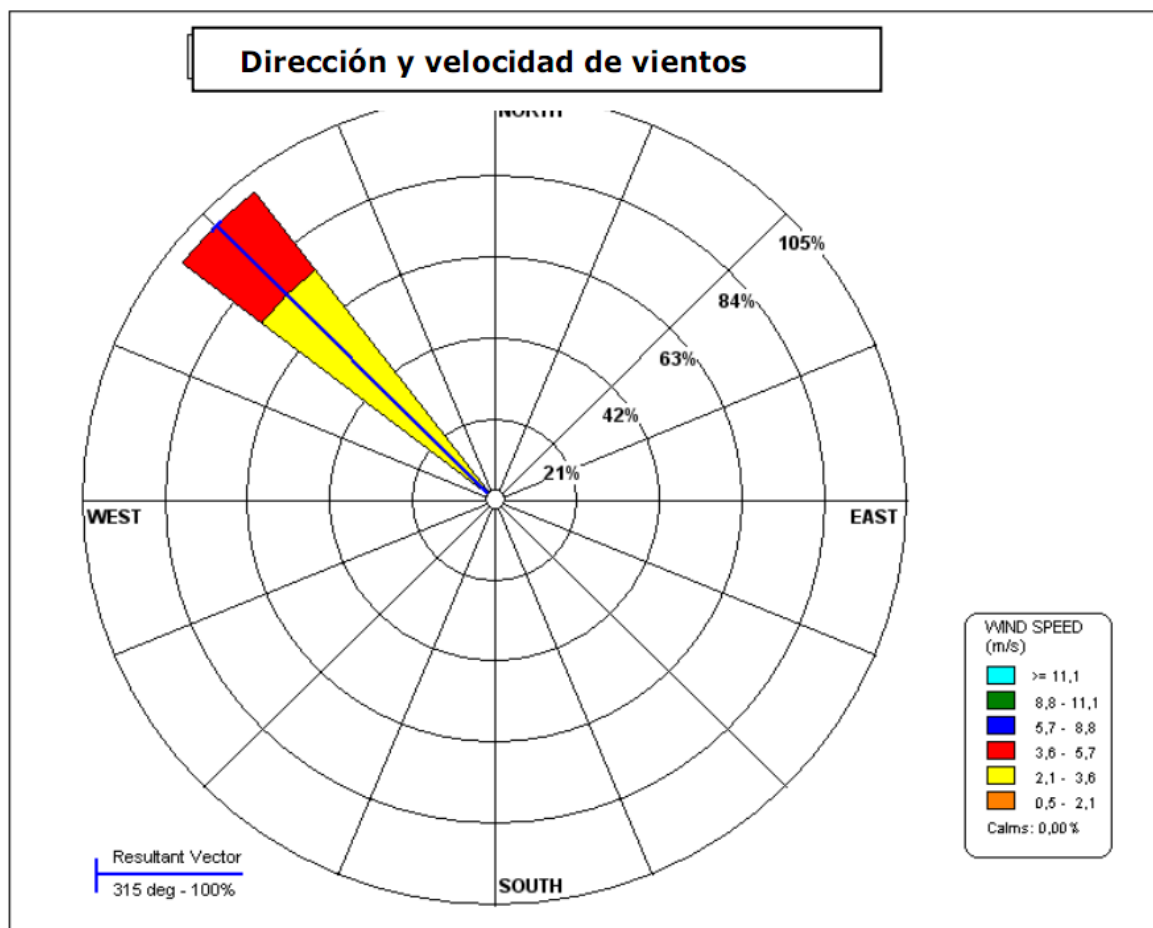
Gráfico 6.6 Rosa de Vientos – Estación Ñaña
