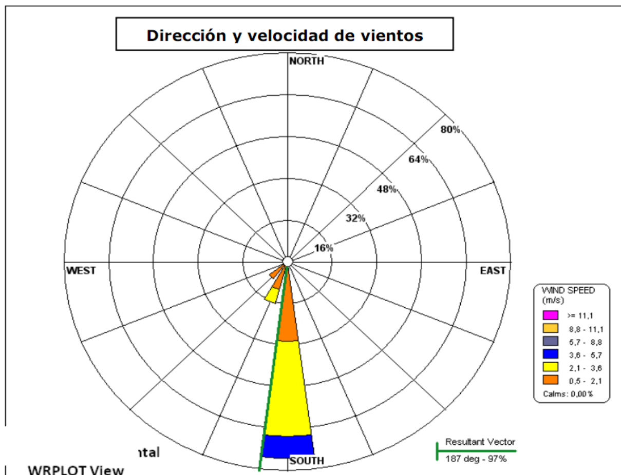
Gráfico 6.4 Rosa de Vientos – Estación Aeropuerto Internacional Jorge Chávez
