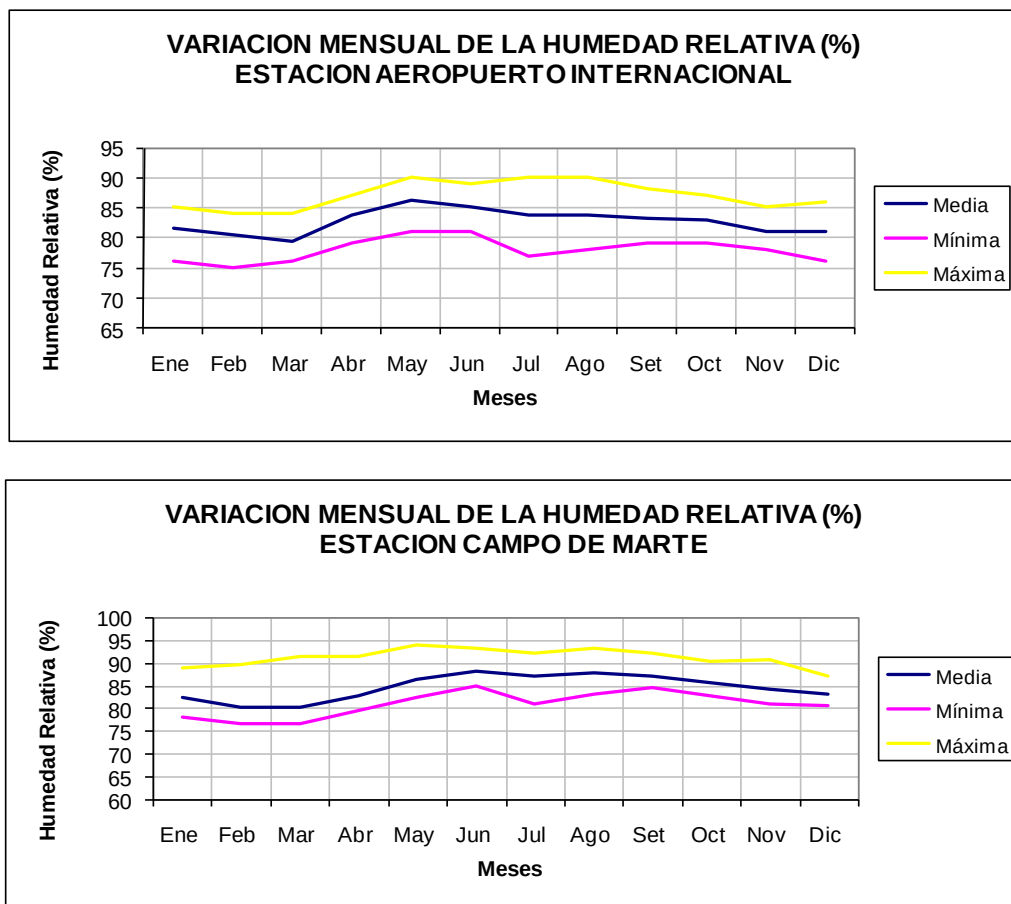
Gráfico 6.2 Variación mensual de la Humedad Relativa
