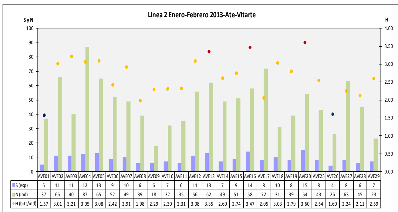
Gráfico 6.11 Análisis de Indicadores de Riqueza (S), Abundancia (N) y Diversidad ( H' ).
