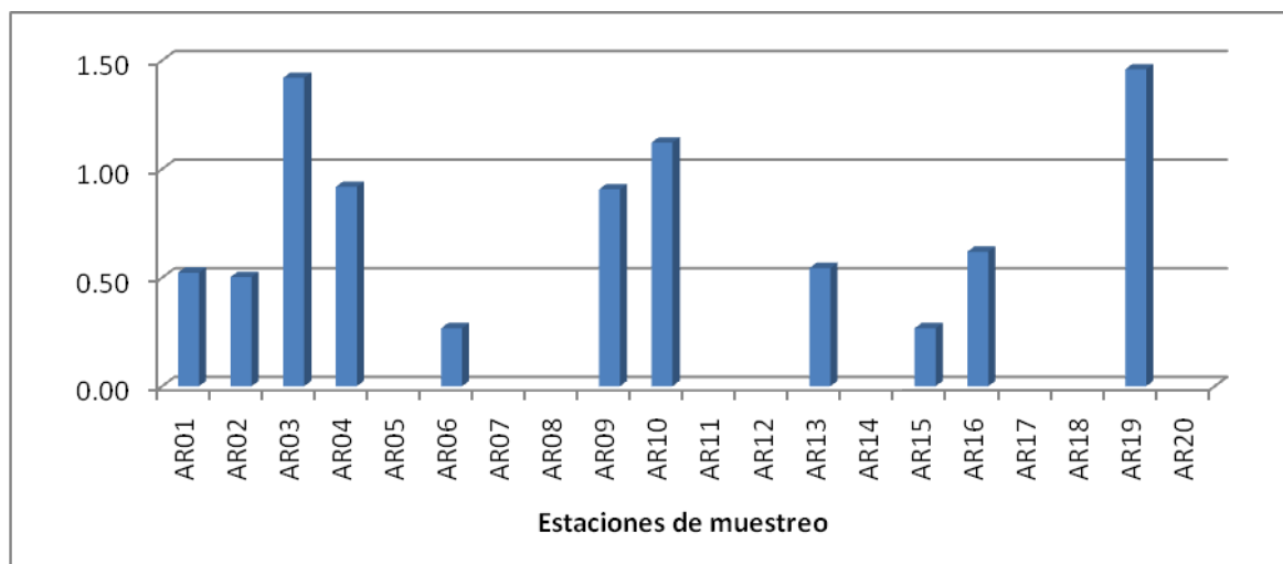
Gráfico 6.47 Análisis de Indicadores de Diversidad (H').
