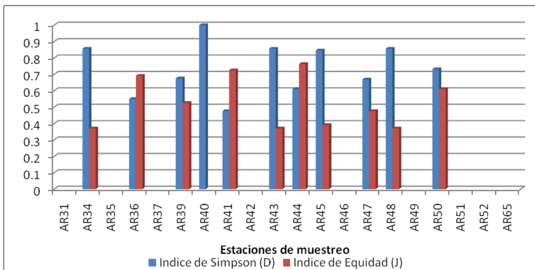
Gráfico 6.38 Análisis de Dominancia (D) y Equidad (J) para puntos con mayor y menor diversidad.
