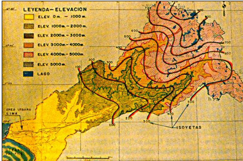
Figura 6.1 Isoyeta de Precipitación Anual – Cuenca del Río Rímac
