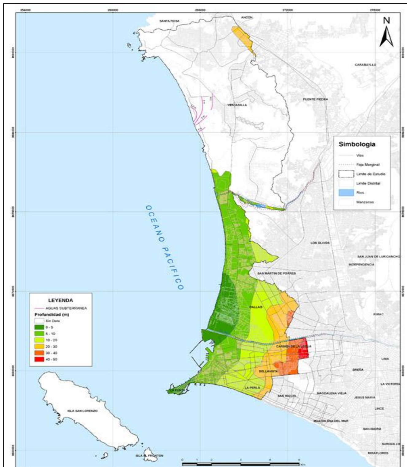
Figura 6.4 Profundidad de aguas subterráneas
