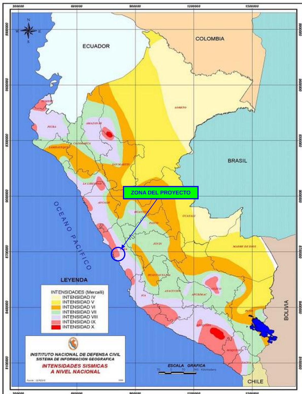
Figura 6.5 Mapa de Intensidades Sísmicas Máximas
