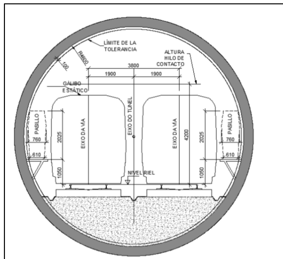
Figura 4-5. Sección circular TBM
