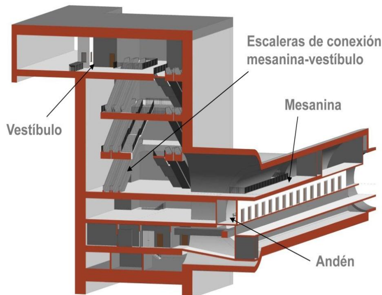
Figura 4-13 3D de la estación tipo caverna
