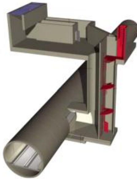
Figura 4-19 Esquema 3D de pozo de ventilación-emergencia
