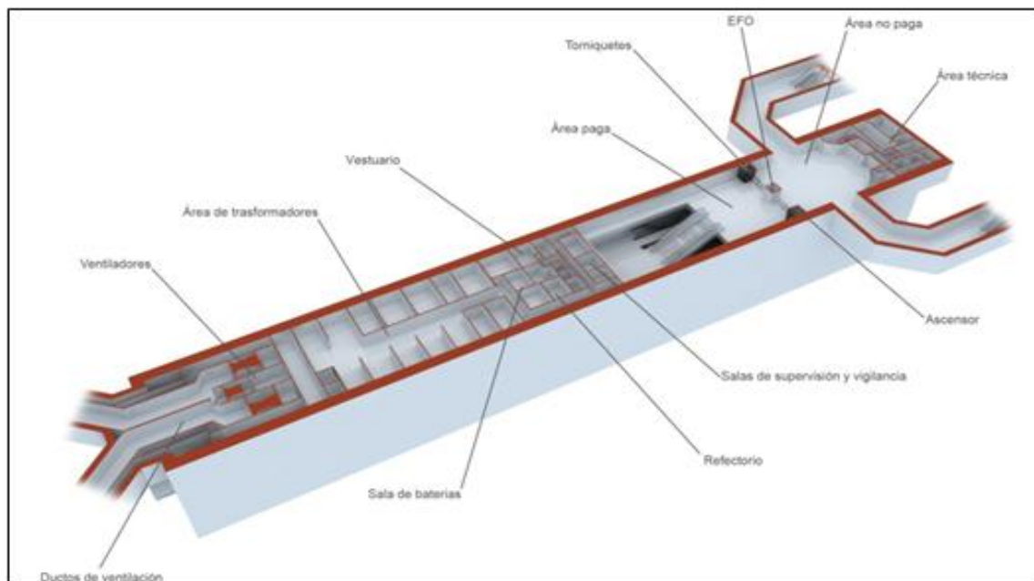
Figura 4-11 Estación Cut&Cover Tipo 1
