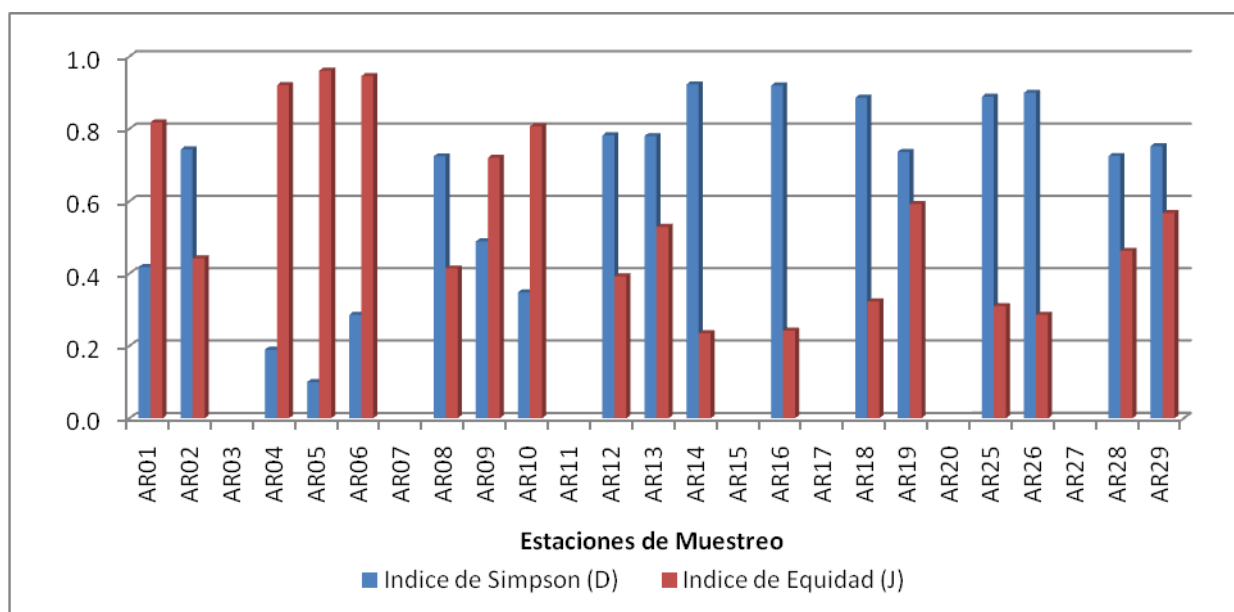
Gráfico 6.32 Análisis de Dominancia (D) y Equidad (J) para puntos con mayor y menor diversidad.
