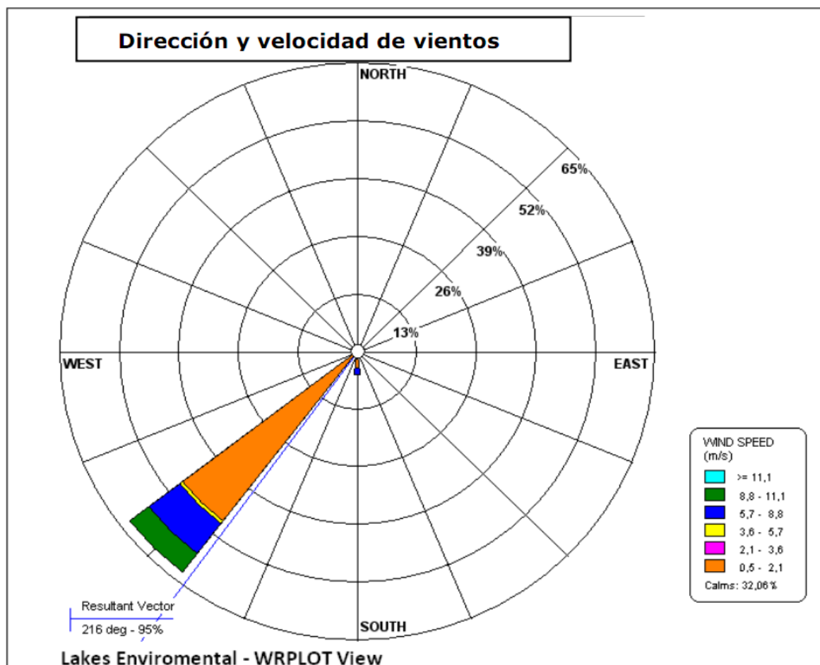
Gráfico 6.5 Rosa de Vientos – Estación Campo de Marte
