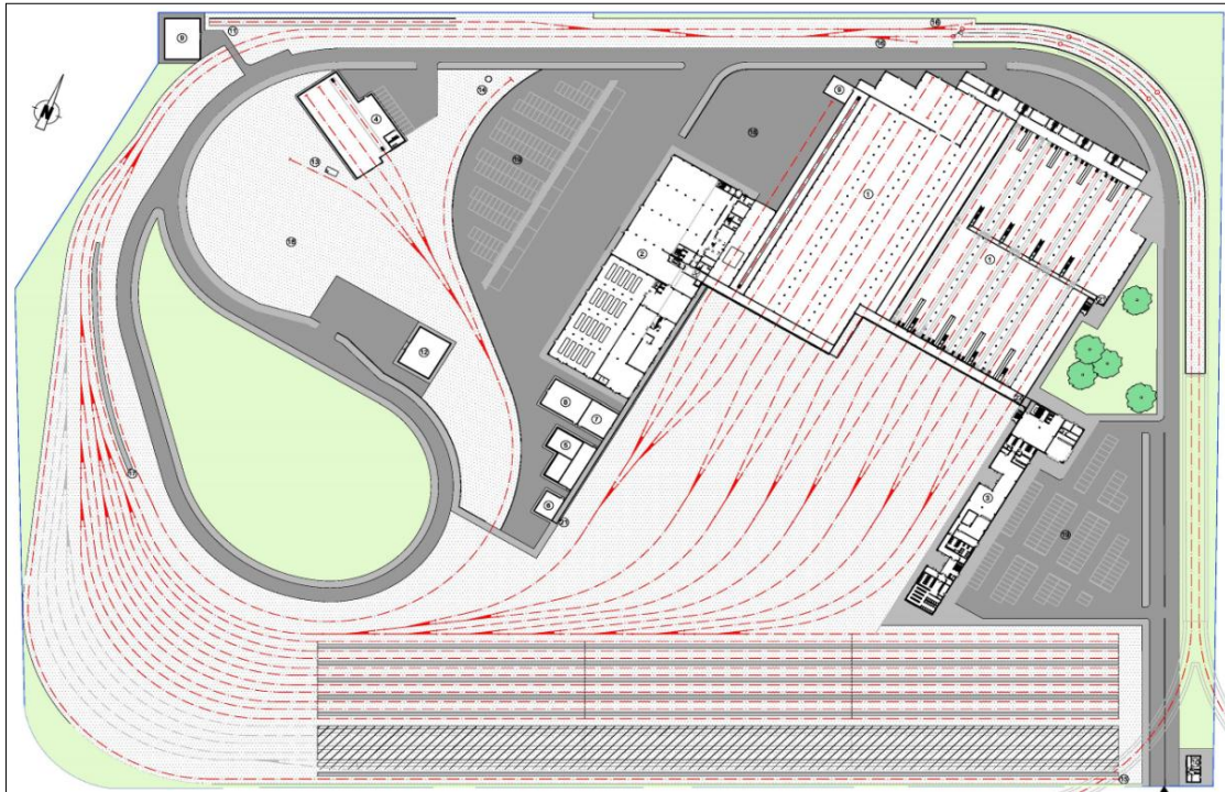
Figura 4-22 Implantación General del Patio Santa Anita
