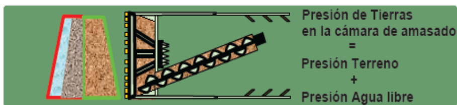
Figura 4-32 Balance de presiones en la cámara de amasado
