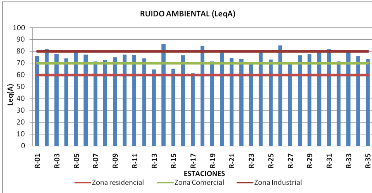
Gráfico 6.7 Resultados de laboratorio – Presión Sonora Ambiental
