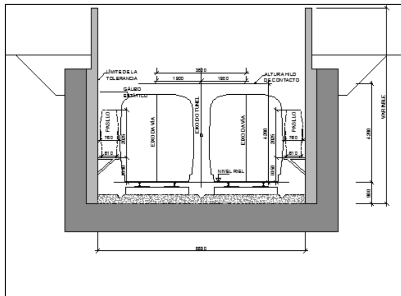
Figura 4-10. Sección rectangular C&C y Trinchera
