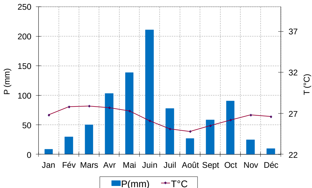
Figure 2 : Courbe ombrothermique de la zone littorale
