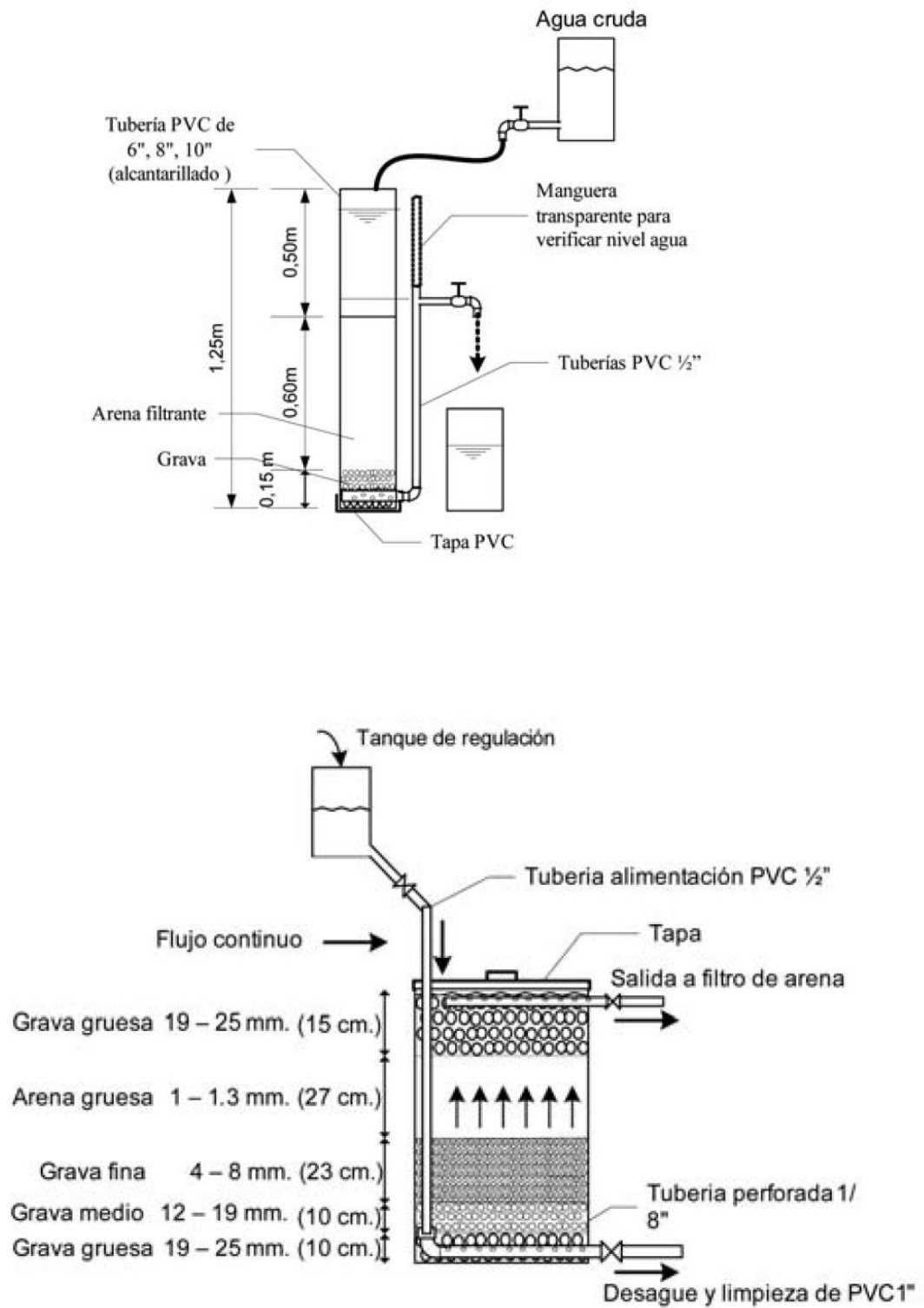
Figura 2 Filtro casero de arena con tubería de PVC
