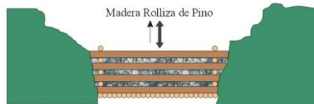
VISTA FRONTAL AGUAS ARRIBA
