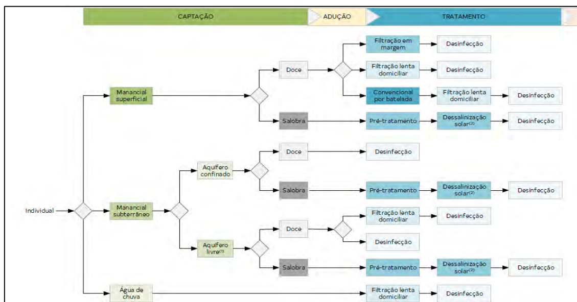
Figura148 – Tipos de Tratamento para Sistema ou Solução de Abastecimento de Água Individual
