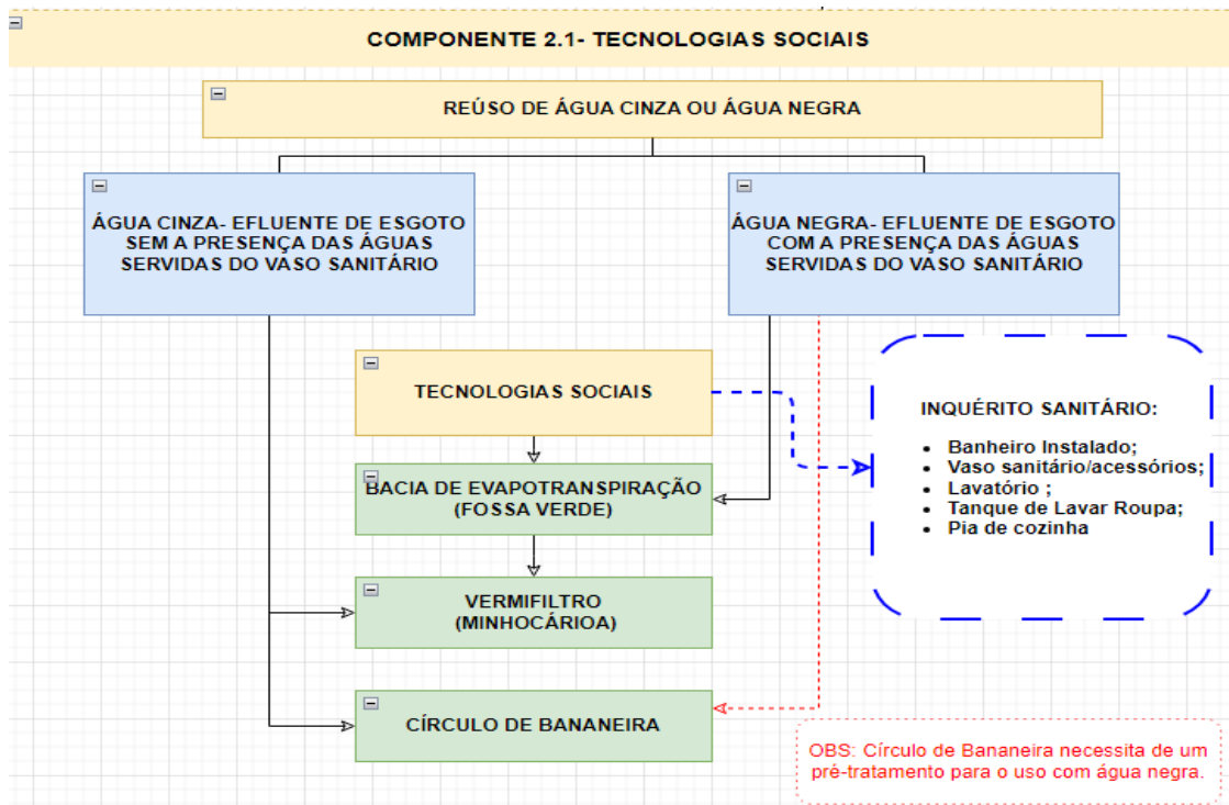
Figura 6 - Diagrama Esgotamento Sanitário e Reuso de Efluente Doméstico Tratado
