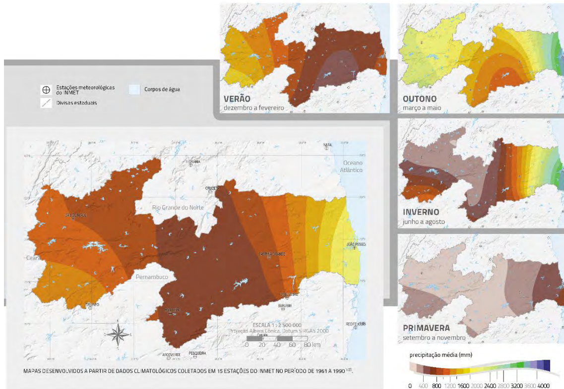
Figura29 – Precipitação Média Anual e Sazonal do Estado da Paraíba
