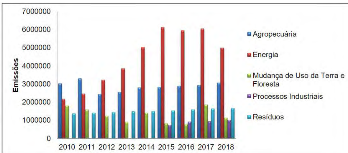
Figura39 – Emissões de GEE por setor em CO 2 e (t) no estado da Paraíba, 2010 - 2018.
