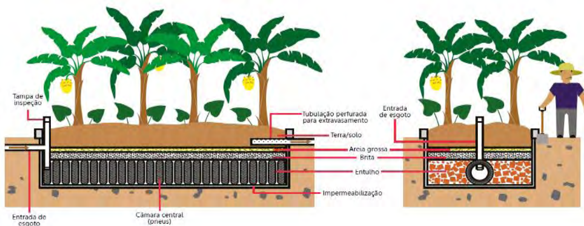
Figura 16 - Bacia De Evapotranspiração (Fossa Verde)
