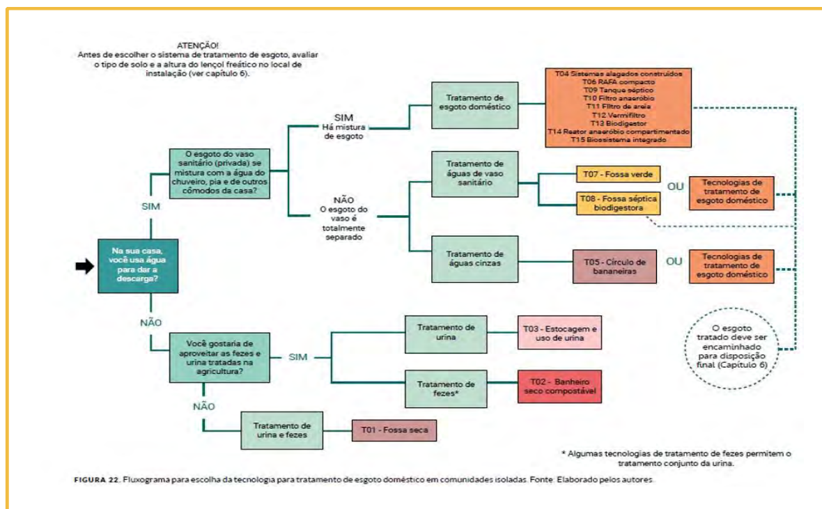
Figura 15 - Tipologias Para Tratamento De Esgoto Em Áreas Rurais
