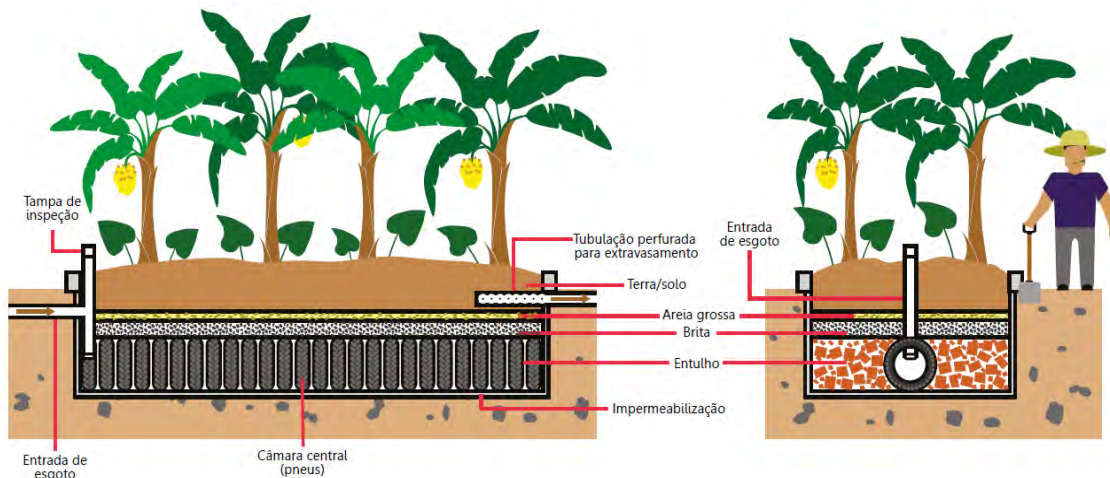
Figura 20 - Fossa Verde - Evapotranspiração
