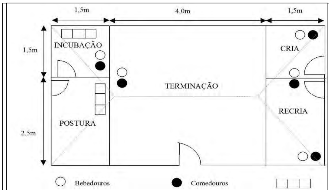
Figura 2 – Croqui ilustrado do projeto
