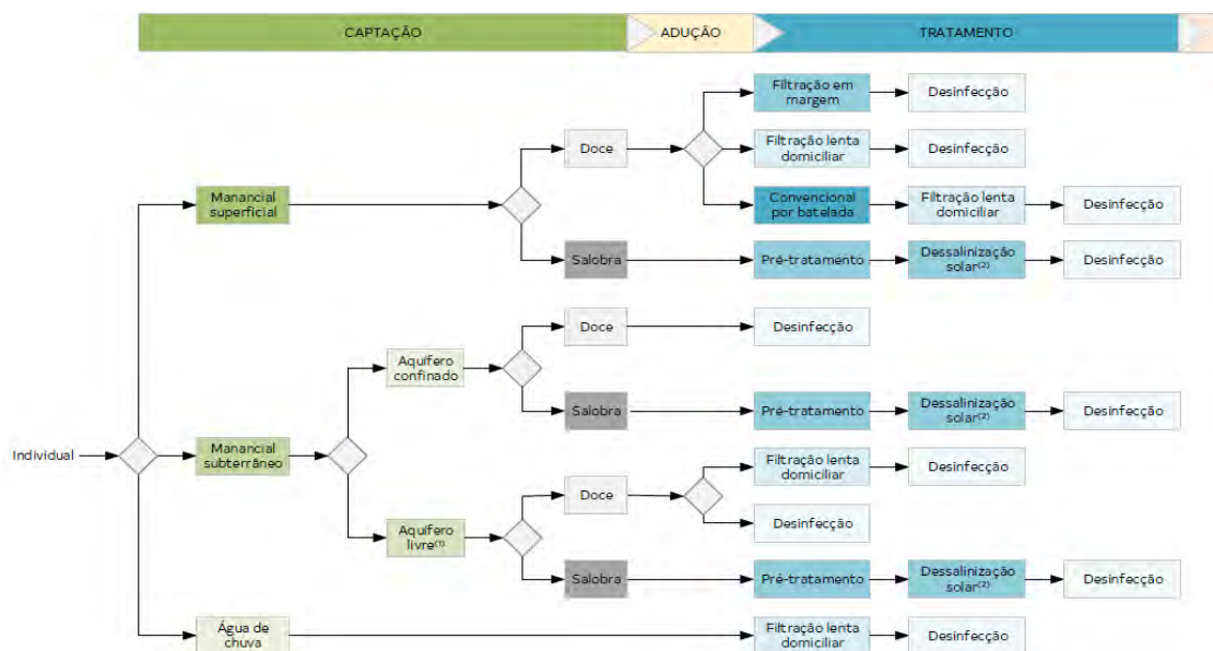
Figura 12 - Tipos De Tratamento Para Sistema Ou Solução De Abastecimento De Água Individual.
