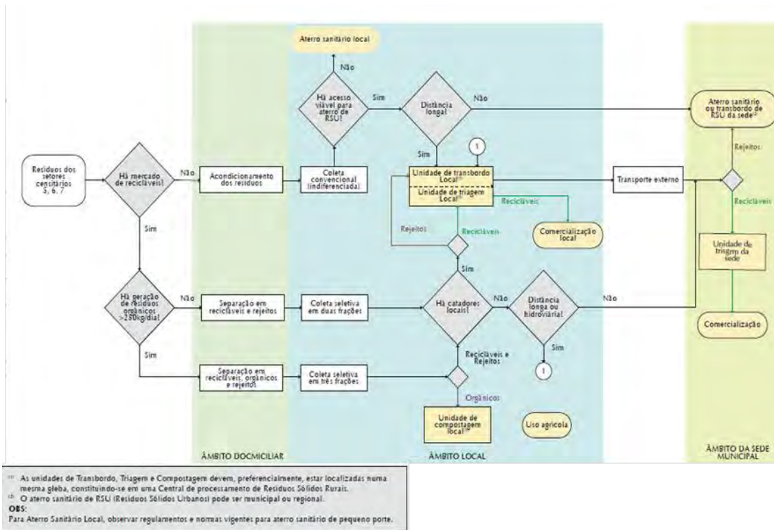
Figura 9 - Matriz Tecnológica de Soluções Coletivas para o Manejo de Resíduos Sólidos
