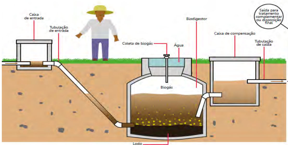
Figura 19 - Biodigestor
