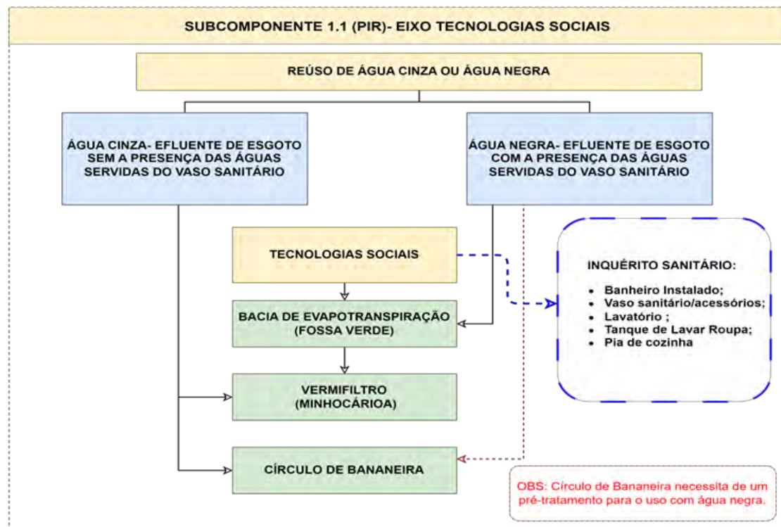
Figura 22 – Fluxograma de Esgotamento Sanitário Reuso de Efluente Doméstico Tratado
