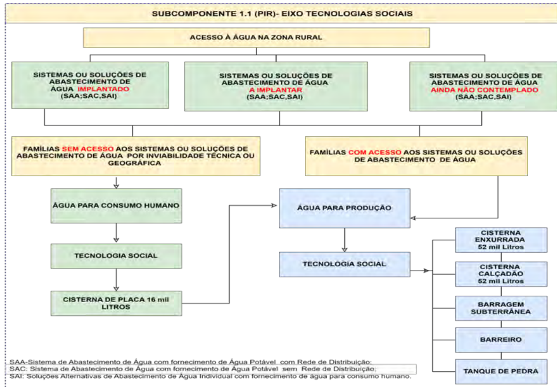
Figura 21 - Fluxograma de definição das Tecnologias Sociais de Abastecimento de Água a serem implantadas
