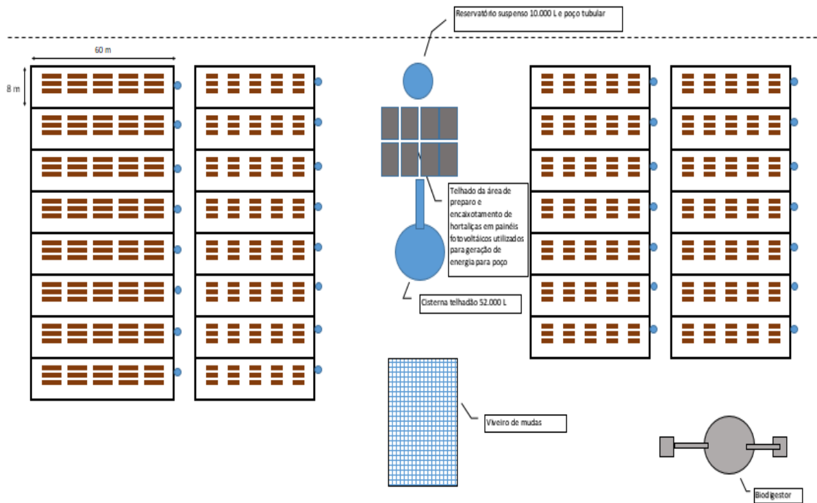
Figura 4 – Croqui dos canteiros
