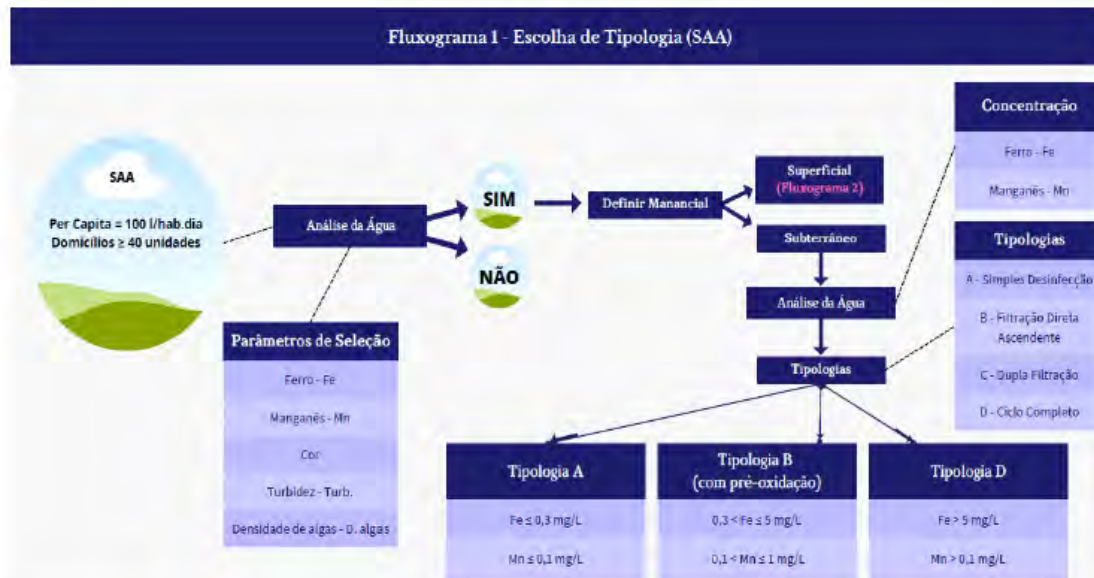
Figura 13 – Fluxograma da escolha de tipologia do SAA para água superficial
