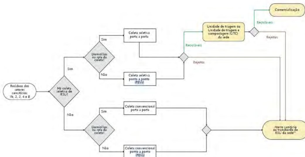
Figura 10 - Matriz Tecnológica de Soluções Coletivas para o Manejo de Resíduos Sólidos com Integração do Sistema Urbano
