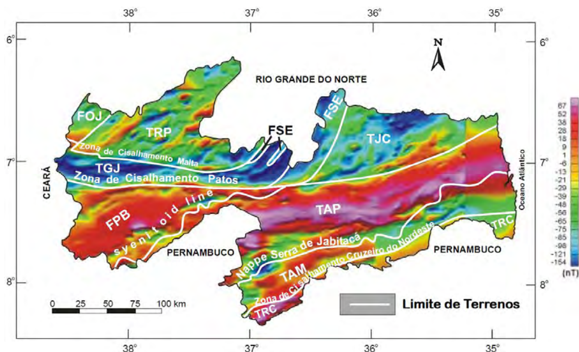
Figura42 – Padrões aeromagnéticos do subsolo paraibano e compartimentação tectono-estratigráfica da Paraíba
