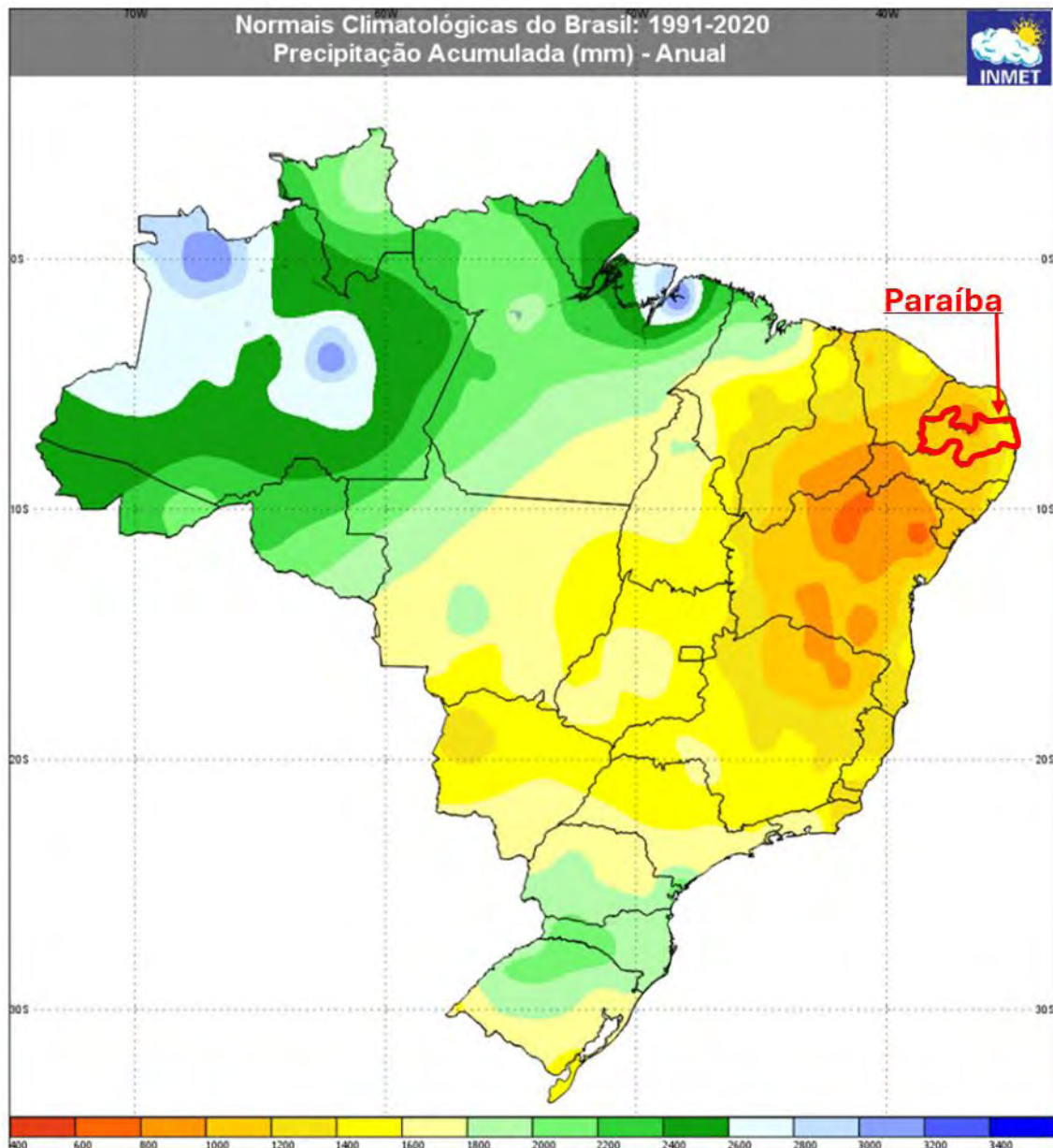
Figura31 – Normal Climatológica do Brasil 1991-2020 – Precipitação Acumulada Anual
