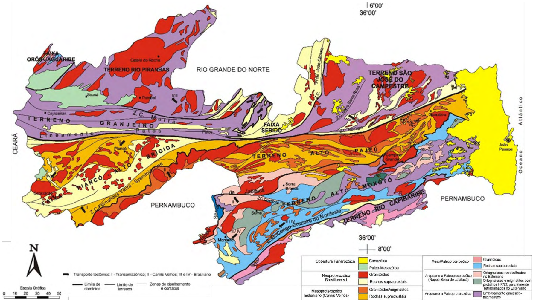
Mapa 1 – Mapa Geológico do Estado da Paraíba
