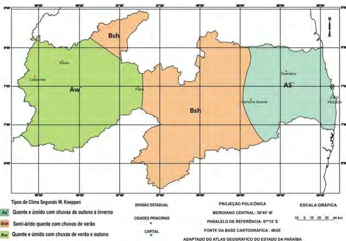
Figura27 – Classificação Climática do Estado da Paraíba – Köppen
