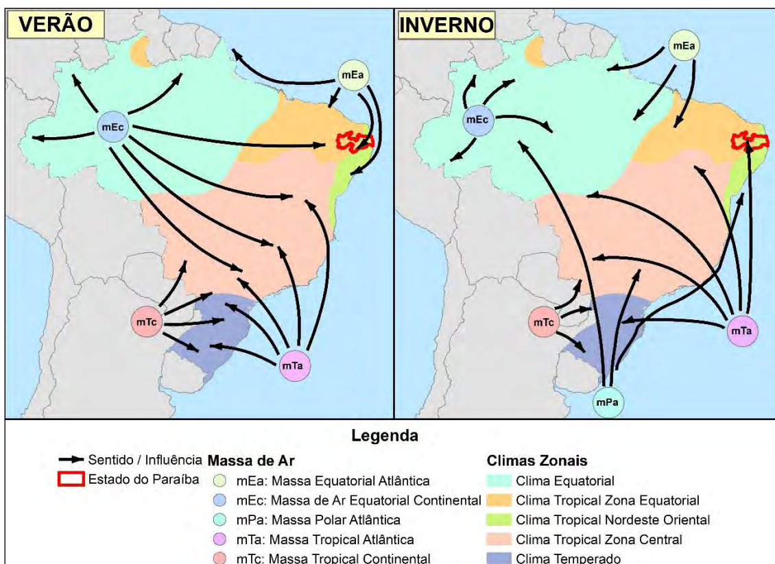
Figura26 – Principais Massas de Ar no Brasil sobre os Climas Zonais
