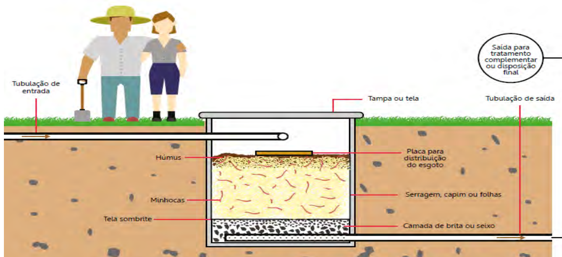
Figura 18 - Vermifiltro
