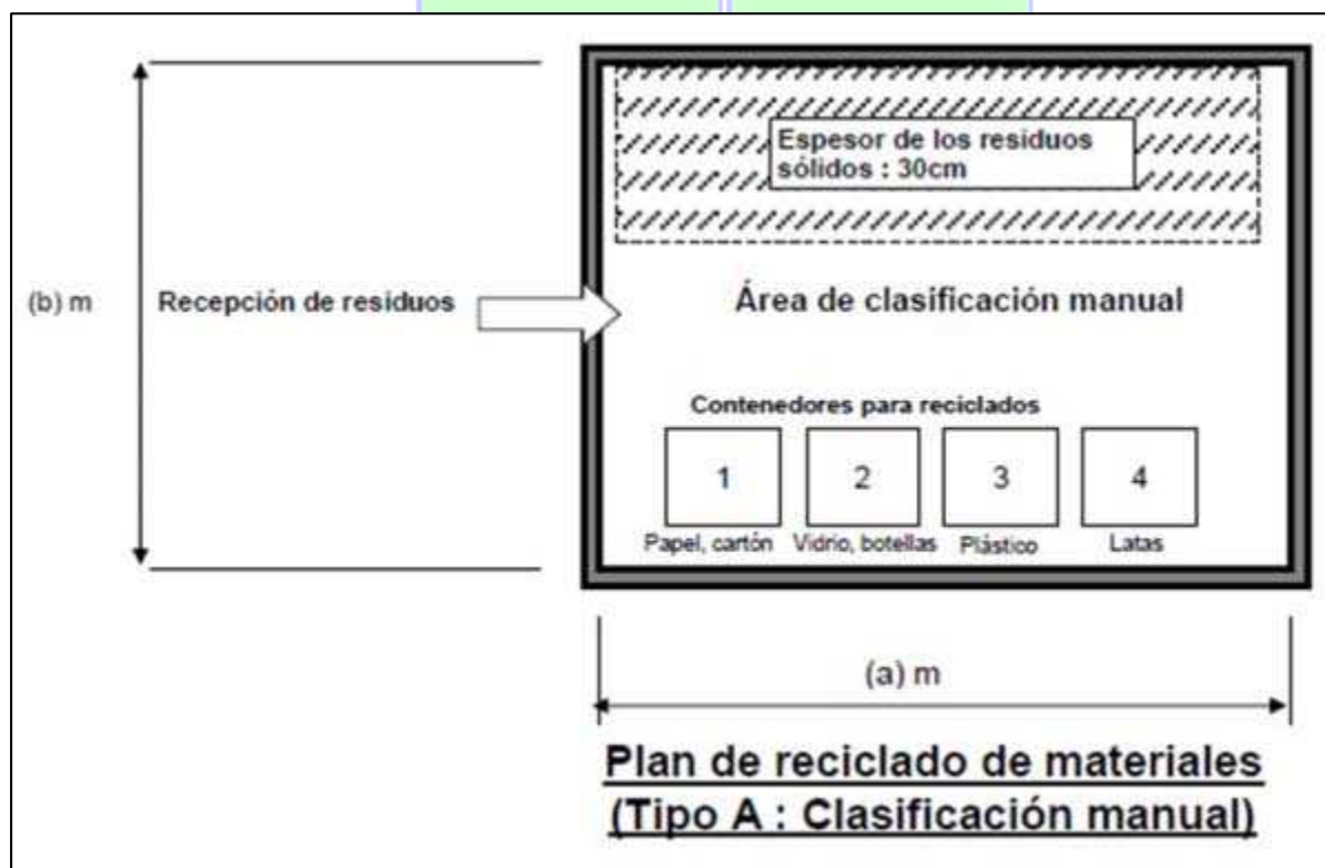
Imagen N° 04: Distribución de planta de Tratamiento de Residuos Sólidos Orgánicos
