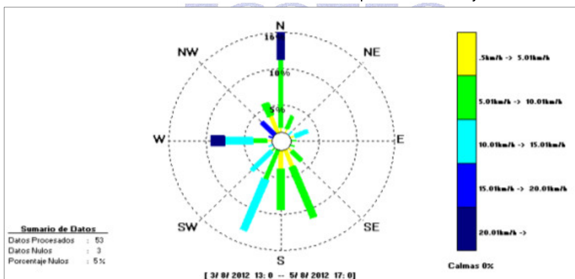
Gráfico N° 04: Rosa De Vientos Para el Área de Emplazamiento Del Proyecto
