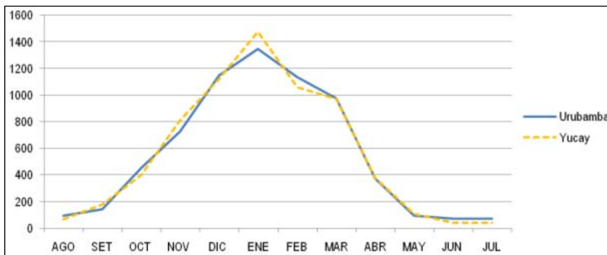
Gráfico N° 01: Precipitación Total Mensual
