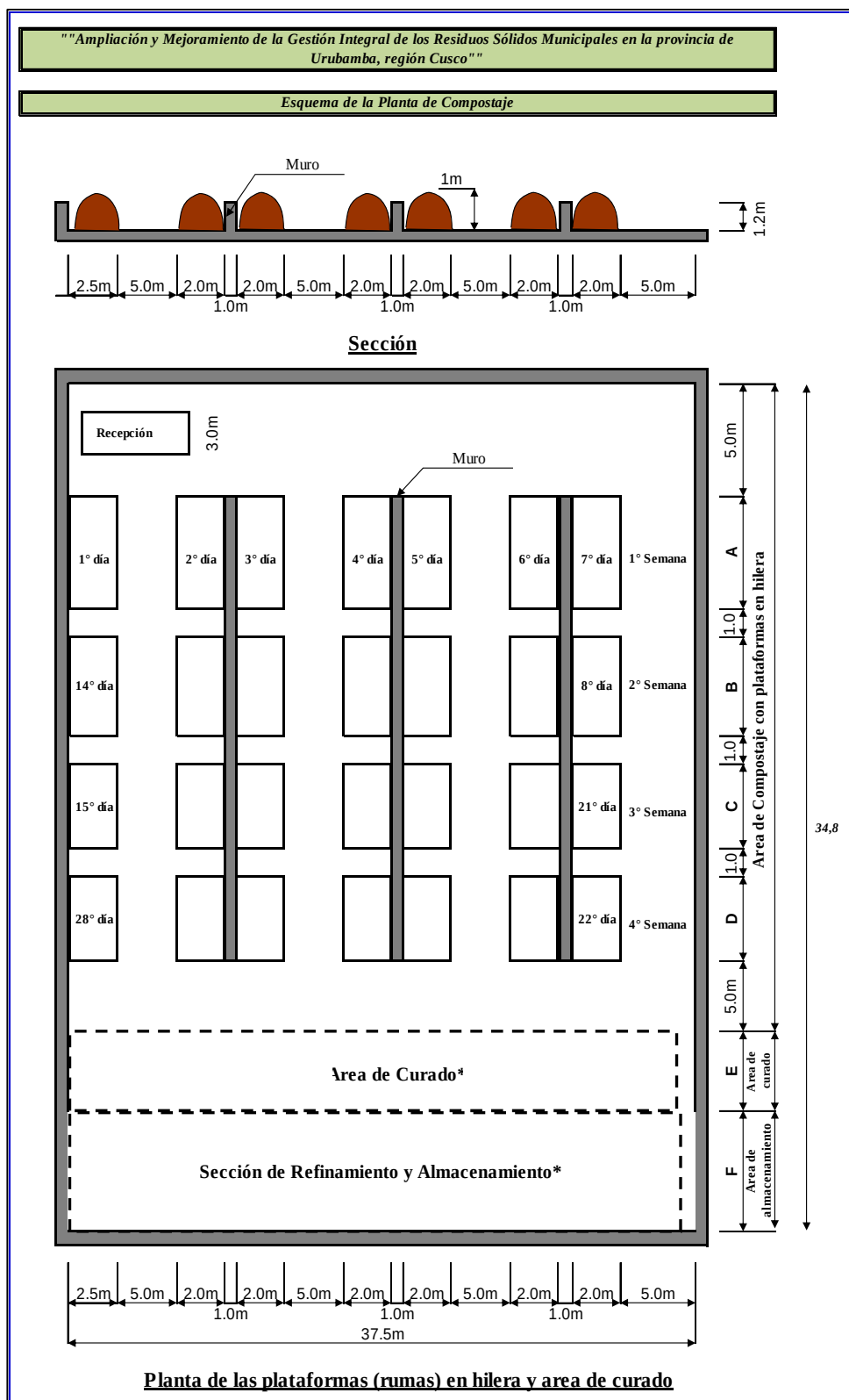
Imagen N° 05: Distribución de la Infraestructura de Aprovechamiento
