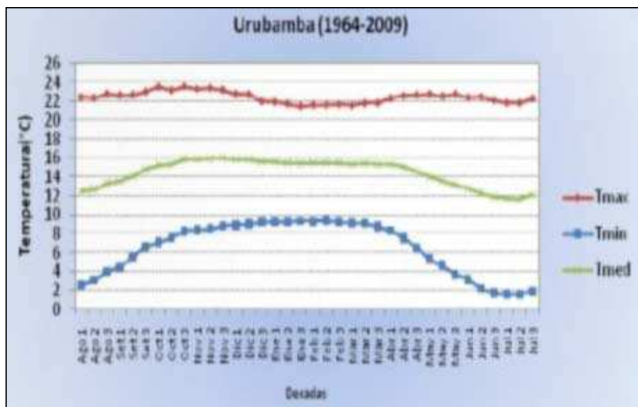
Gráfico N° 03: Comportamiento de la Temperatura Máxima, Mínima y Media – Estación Urubamba
