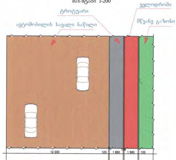
ზ.ჭავჭავაძის ქუჩის მონაკვეთის გეგმა
