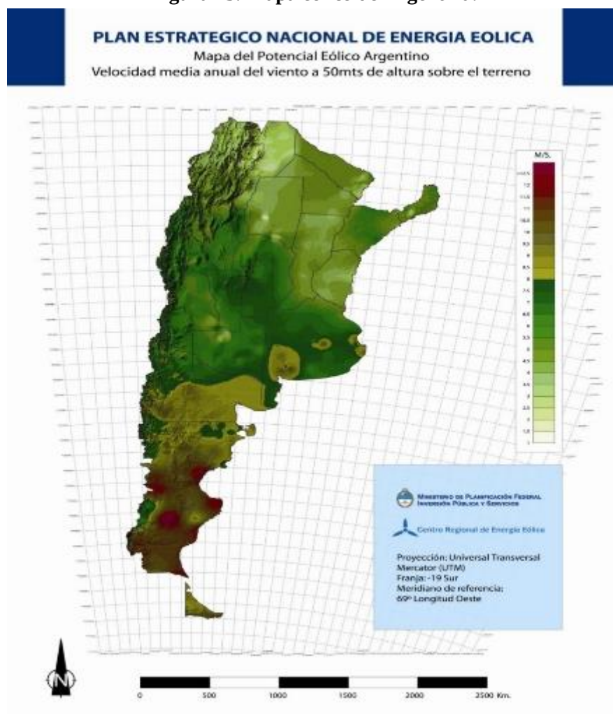
Figura 13. Mapa eólico de Argentina.
