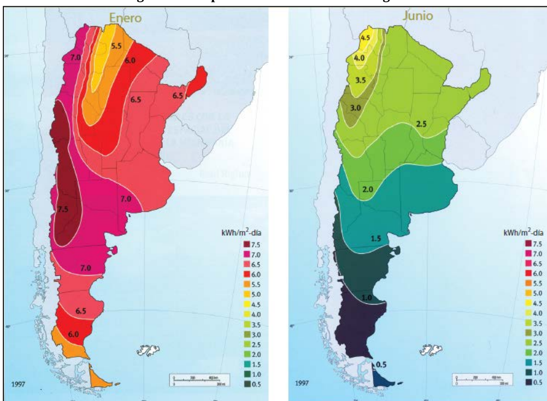
Figura 14. Mapas de radiación solar en Argentina.
